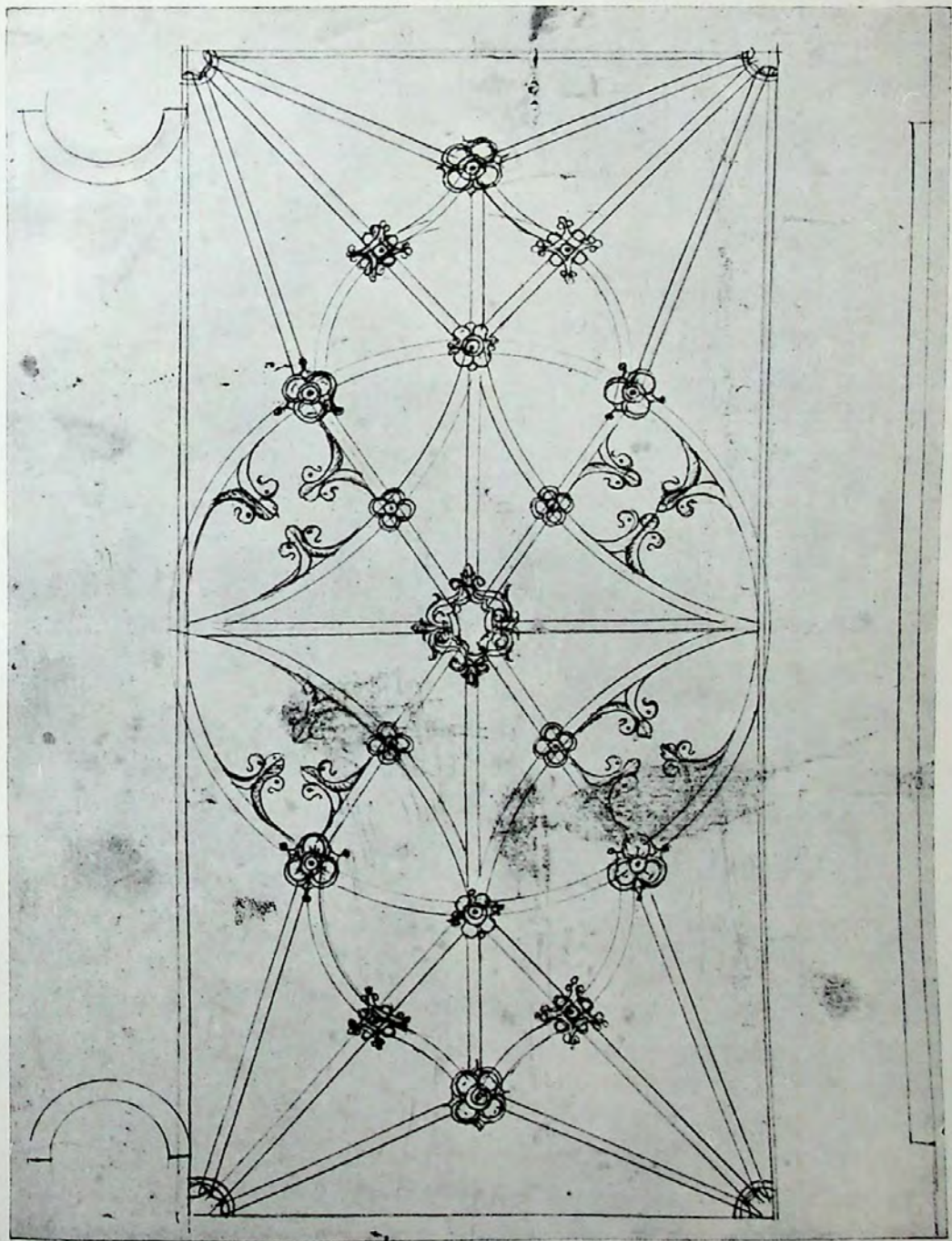
LÁMINA IV. —Castromocho. San Esteban. Capilla del bachiller Juan Rodríguez. Trazo de las bóvedas por Gaspar de Solórzano.
