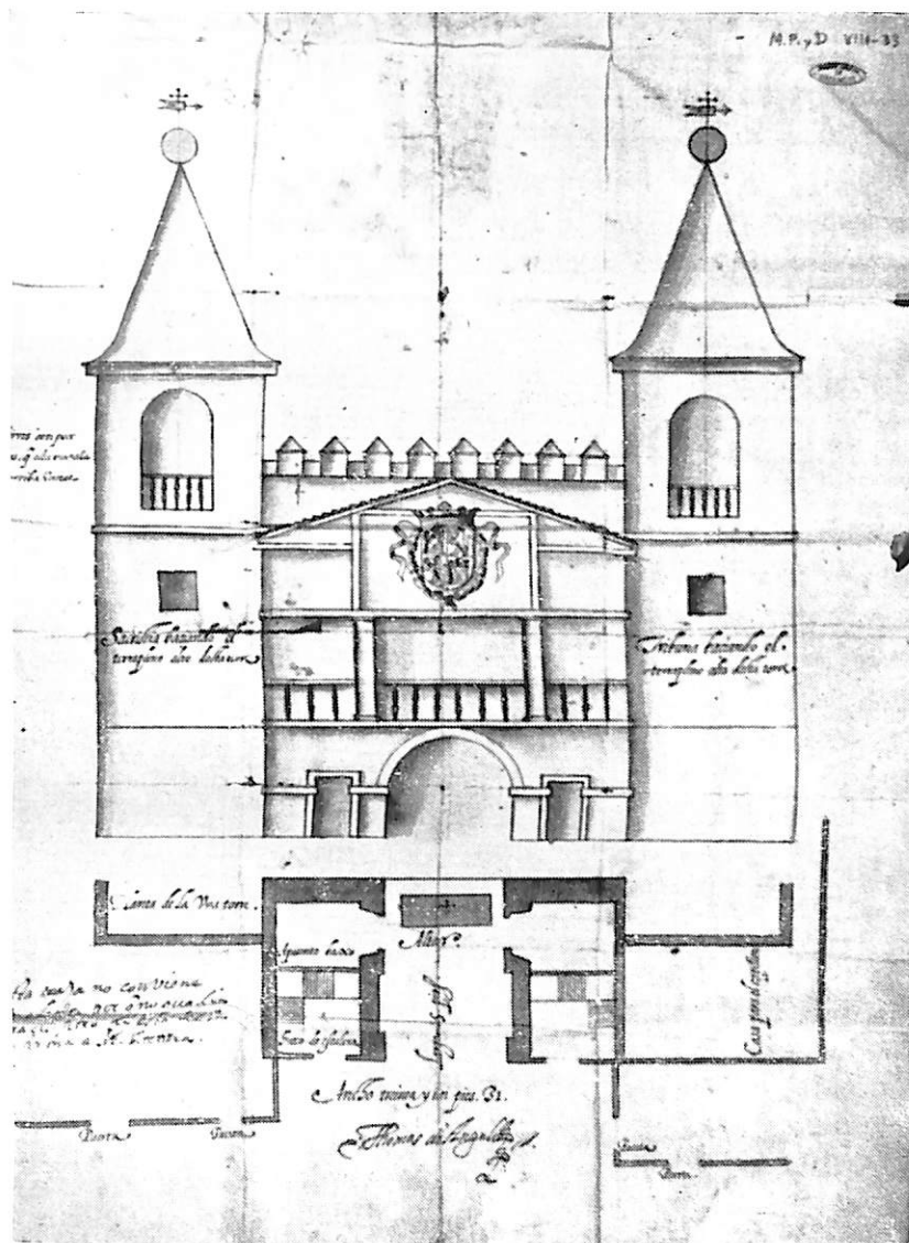
Fachada y planta para la nueva capilla de Nuestra Señora del Populo de Cádiz (1618).
