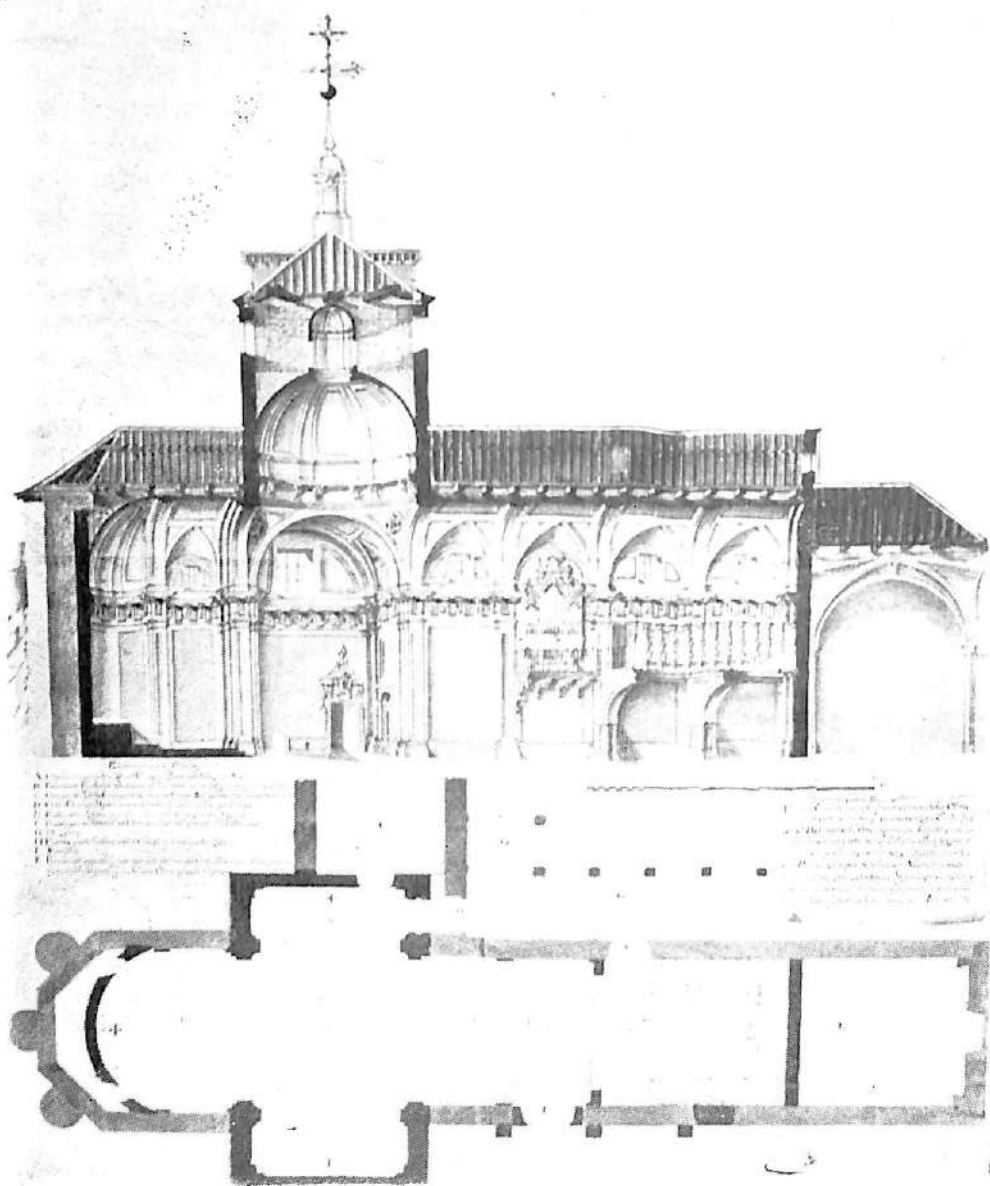
Planta, elevación y corte de la Iglesia de San Bernardo, extramuros de Toledo. Núm. 160, anexo.
