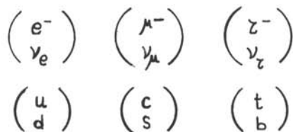
As tres xeracións de leptóns e quarks. FIG. 2
