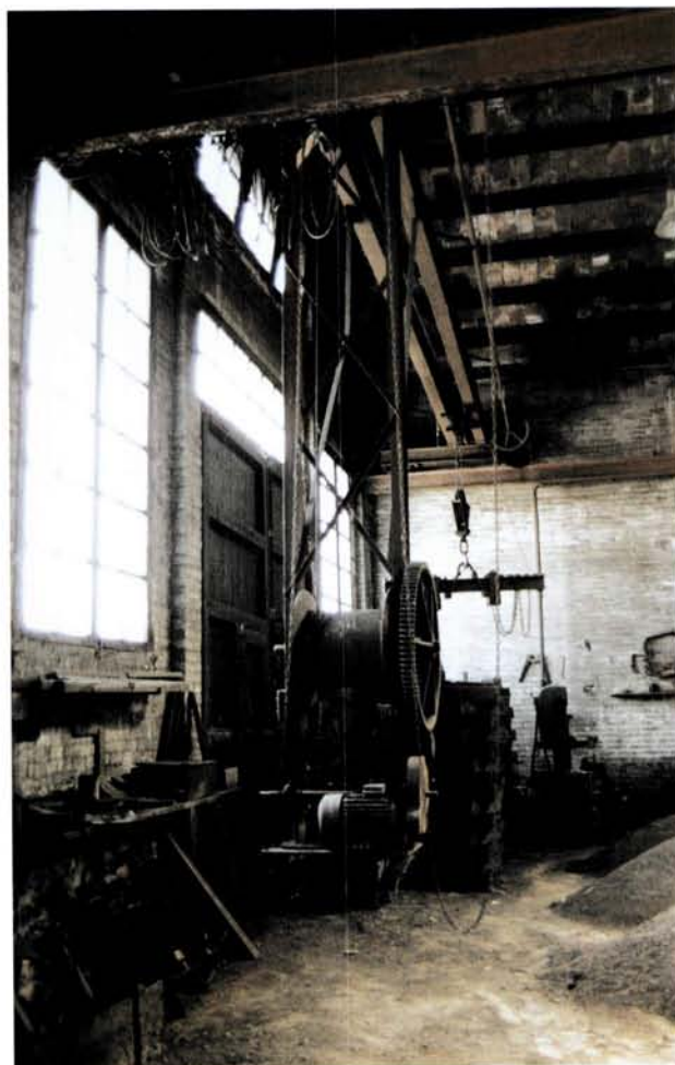
Nau número 1. Màquina de fer motlles amb resines sintètiques. Any 1995. (Fotografia: Oriol Saula. AFMCUT)
