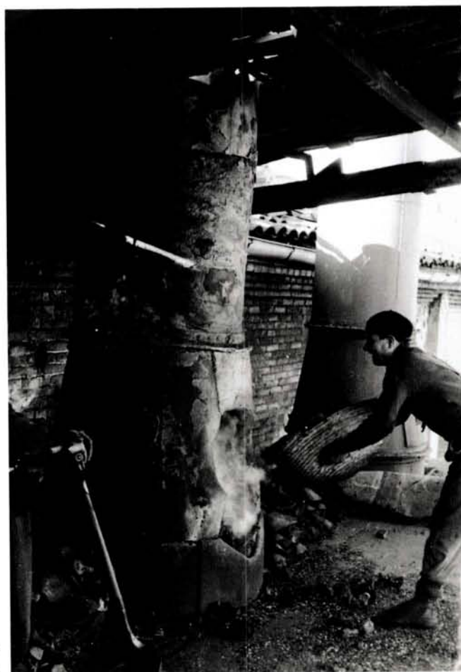
Secció de foneria, càrrega del cubilot. Anys 50. (Arxiu de les indústries J. Trepal)
