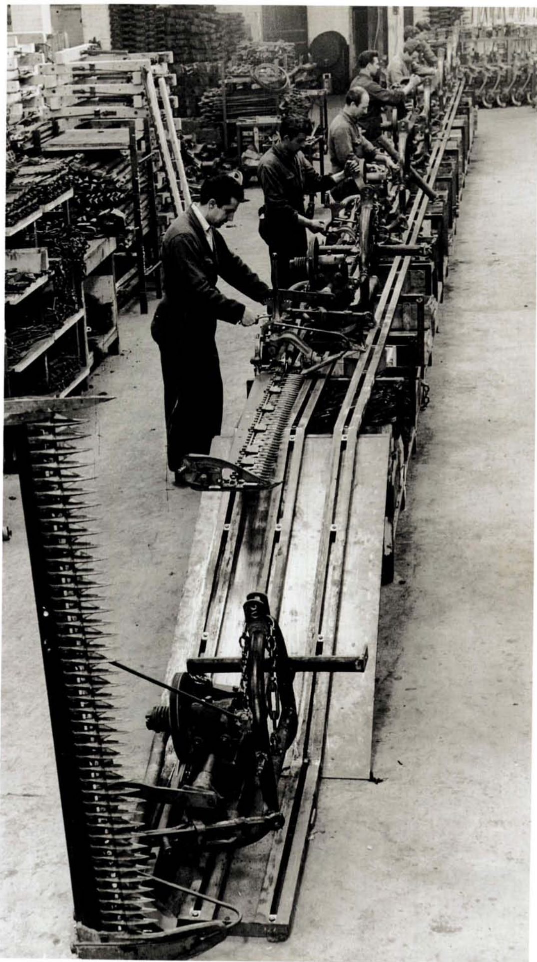
Nau número 9. Els treballadors de la cadena en ple muntatge de les màquines segadores d'alfals per a tractor. Anys 1961-62. (Fotografia: Calafell. Arxiu de les Indústries J. Trepal)
