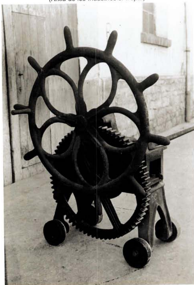
En aquestes tres imatges veiem una màquina de foradar, una màquina de corbar i una màquina de recalcar. Aquestes tres màquines es van produir a la fàbrica J. Trepat per a ús propi, però posteriorment es van comercialitzar per als ferrers i els representants que l'empresa tenia per tot el país. (Arxiu de les Indústries J. Trepat)
