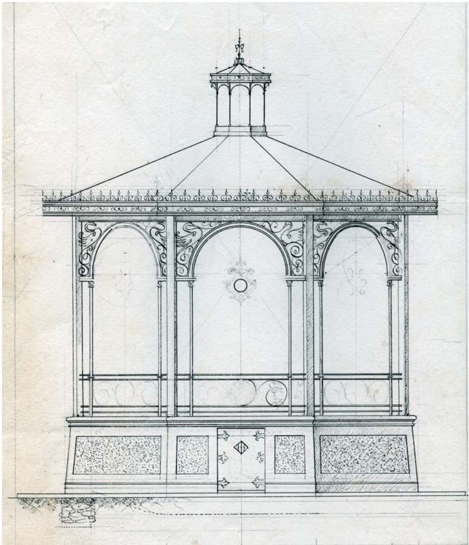
Borrador de kiosko da Banda de Música. (arredor de 1913). AMB, c-7742.
