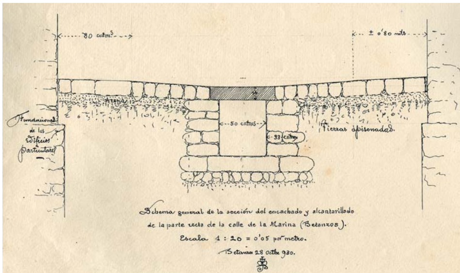
Plano de sección de encachado e alcantarillado da parte recta da rúa da Marina. 1930. AMB, c-3437.
