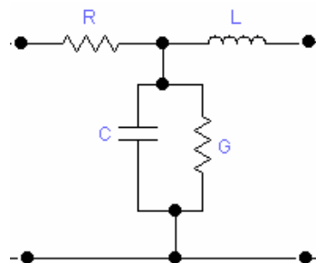
Figura No. 3. Constantes eléctricas primarias por unidad de longitud
