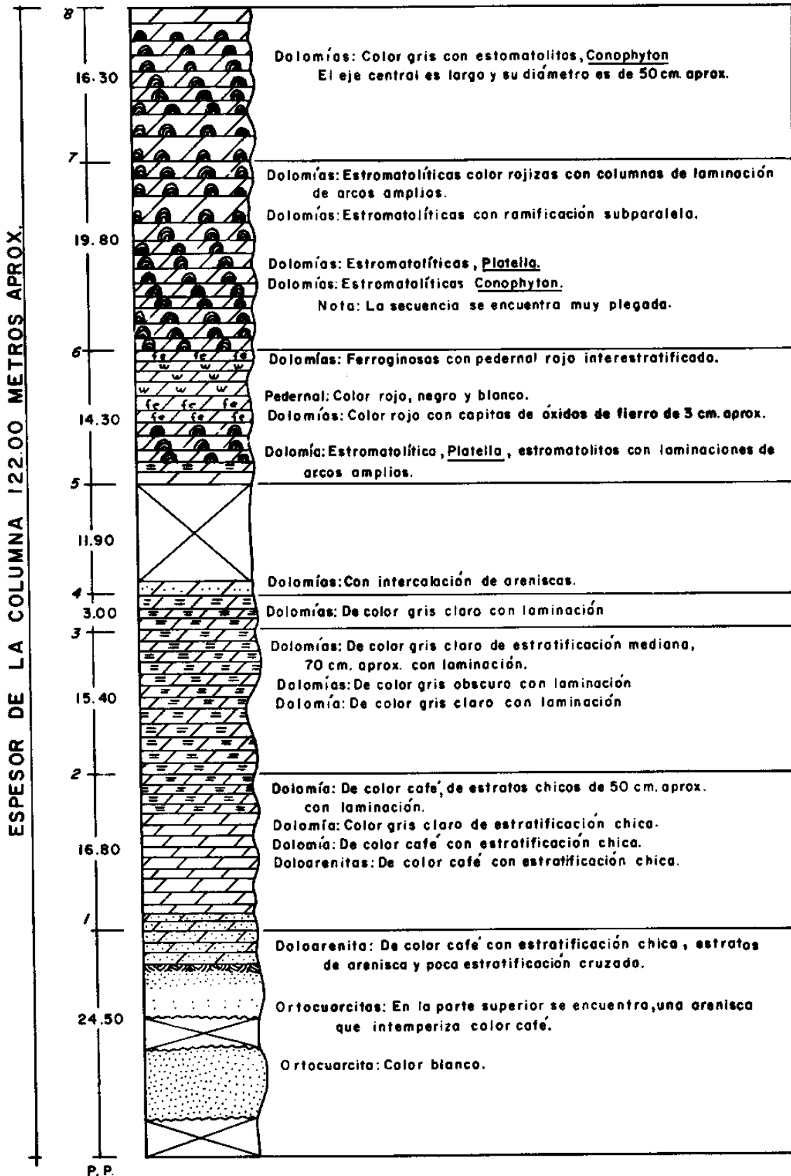
Figura 7.- Sección columnar que ilustra la secuencia litológica y nivel con contenido estromatolítico en los cerros al NW de La Ciénega. Nótese la presencia de pedernal en la unidad que contiene estromatolitos.
