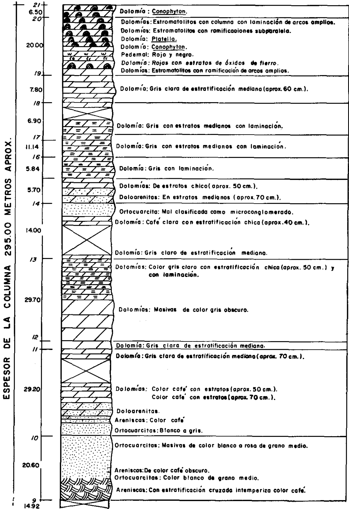
Figura 6.- Sección columnar que ilustra la secuencia litológica y nivel con contenido estromatolítico en el Cerro Clemente. Nótese la presencia de pedernal en la unidad que contiene estromatolitos (continuación).
