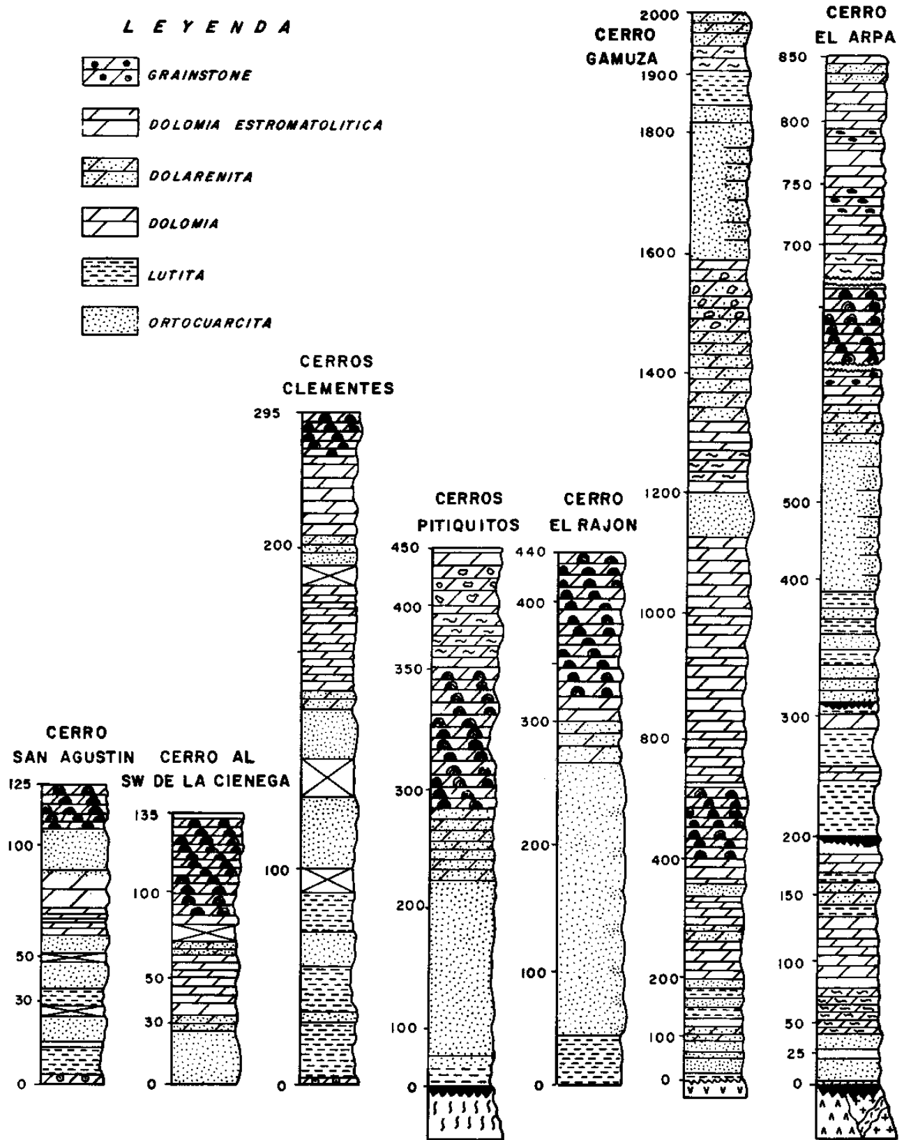
Figura 2.- Columnas estratigráficas levantadas en diferentes localidades precámbricas. Las señaladas bajo el nombre de Cerro San Agustín, cerro al SW de La Ciénega y Cerros Clemente, corresponden al presente estudio. La referida como Cerros Pitiquito es de Mendoza (1979), el Cerro Rajón es de Longoria y Pérez (1978), los Cerros Gamuza y Cerros El Arpa son de Longoria y González (1979). No se incluye la columna de Eells (1972) por ser compuesta, aunque básicamente consistiría en sobreponeer cualquiera de las tres columnas introducidas en este trabajo en alguna de las otras columnas presentadas.
