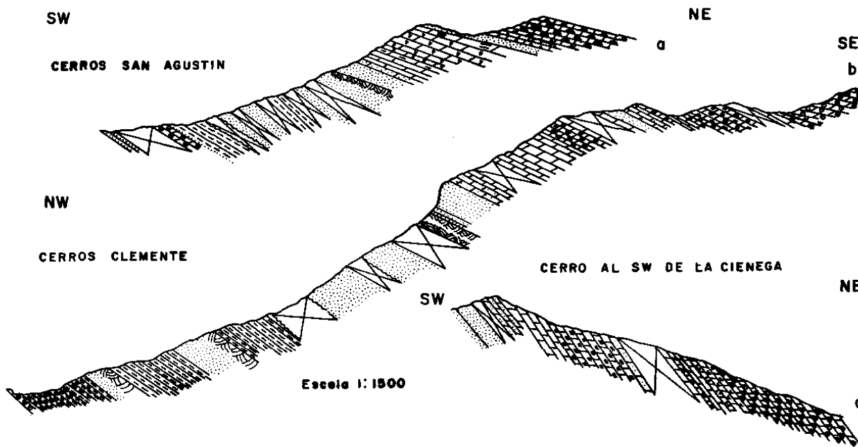
Figura 3.- Perfil esquemático de las tres localidades estudiadas con detalle en este trabajo.
