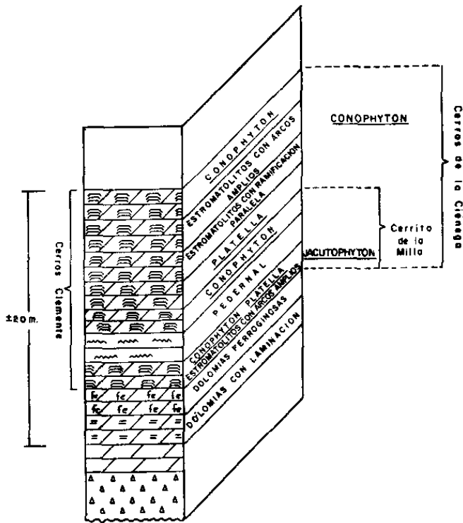
Figura 5.- Sección columnar que ilustra la secuencia fosilífera de la Formación Gamuza en las localidades aquí presentadas. Los tipos estromatolíticos son distintos a los reportados previamente en la literatura e indican un cambio de facies.
