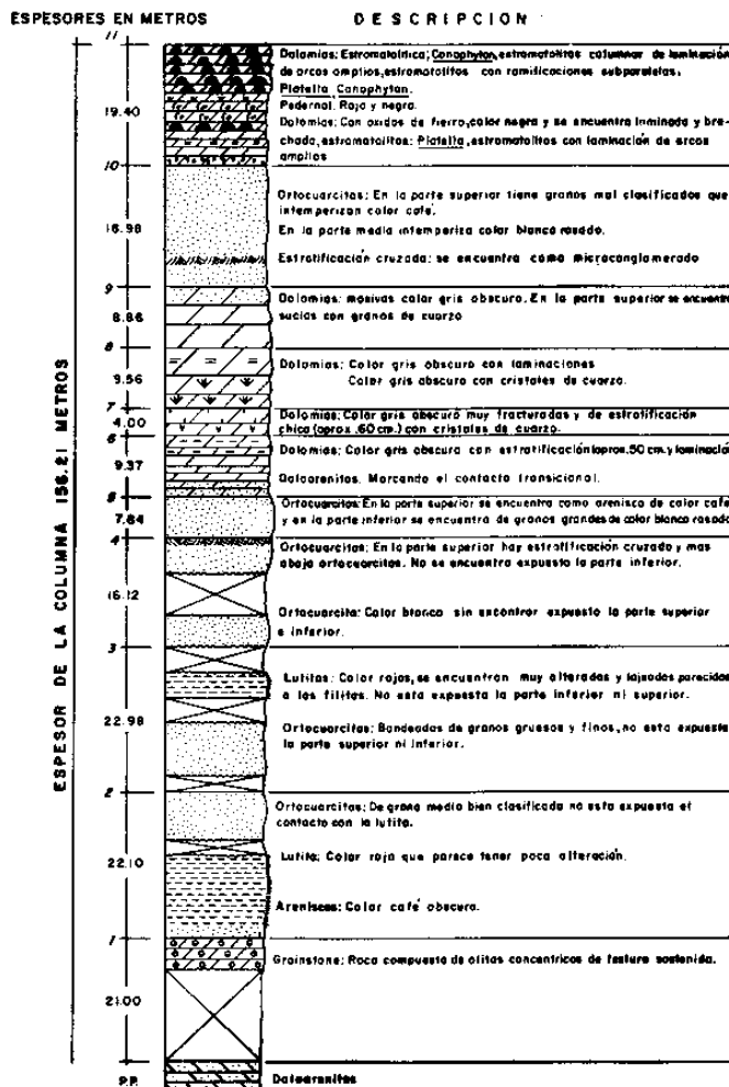
Figura 4.- Sección columnar que ilustra la secuencia litológica y nivel con contenido estromatolítico en los Cerros San Agustín. Nótese la presencia de pederzal en la unidad que contiene estromatolitos.
