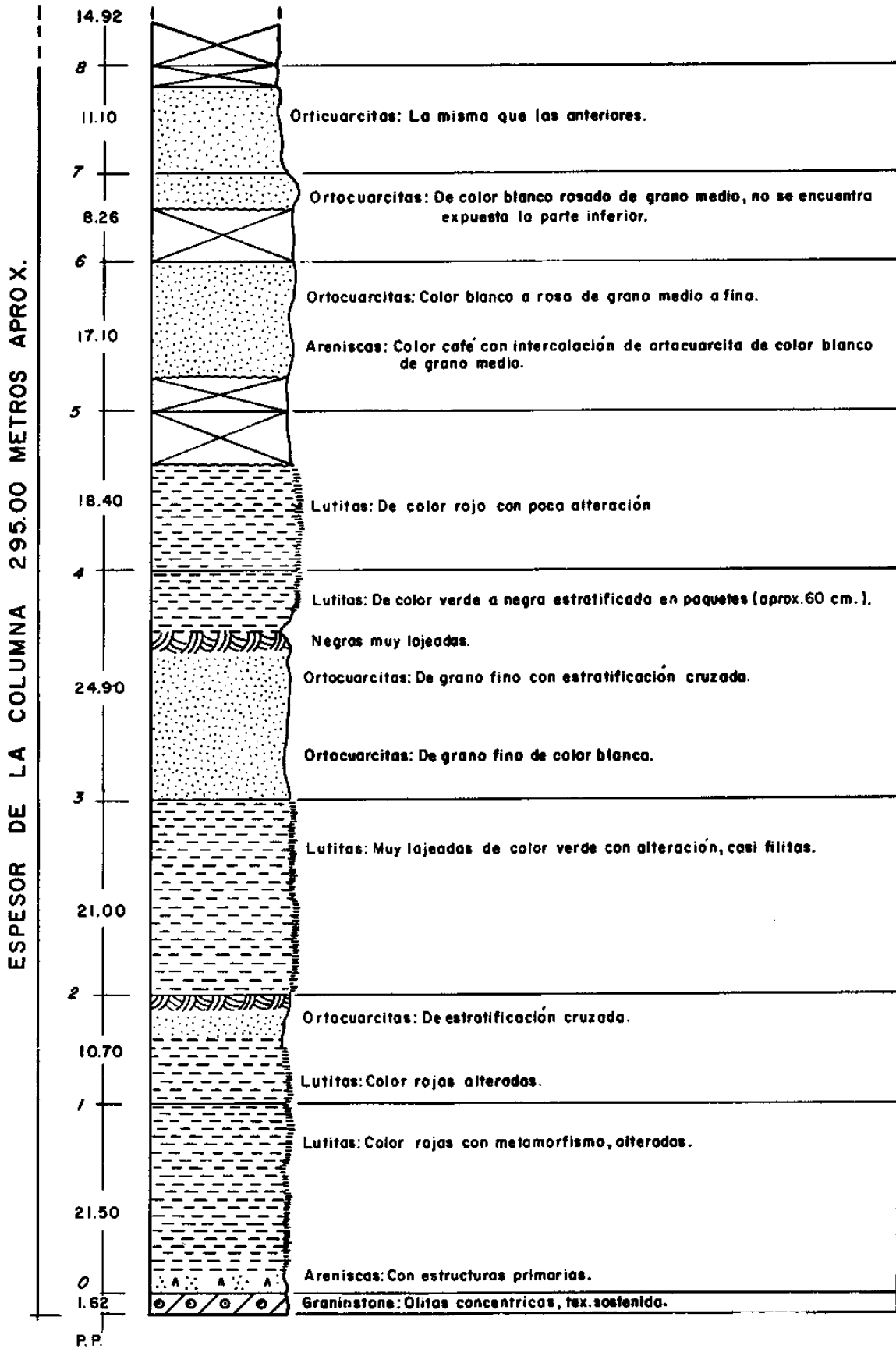
Figura 6.- Sección columnar que ilustra la secuencia litológica y nivel con contenido estromatolítico en el Cerro Clemente. Nótese la presencia de pedernal en la unidad que contiene estromatolitos.
