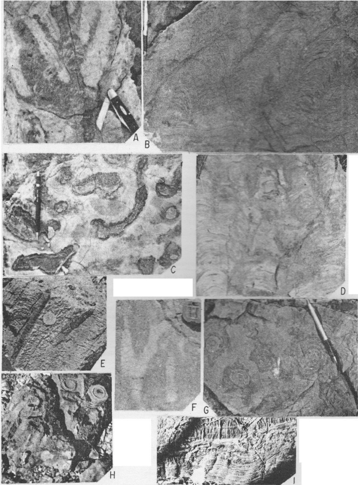
Figura 8.- Estromatolitos de Caborca, Sonora. (A) Estromatolito columnar ramificado del tipo Jacutophyton descrito por Weber y colaboradores (1979) en la Sierra del Viejo. (B) Estromatolitos columnares del tipo Conophyton desarrollado a partir de un estromatolito estratiforme en la Sierra del Viejo, pertenece a la transición de la Formación Pupalote y Formación Llano Verde. (C) Estromatolitos en forma de plancha (tablas) del tipo Platella en los Cerros de La Ciénega desarrollándose libremente, éstas son las ramas del Jacutophyton descrito por Cevallos y Weber (1980). (D) Estromatolitos con ramificación subparalela en el Cerro Clemente. (E) Zona axial de un Conophyton reemplazado en los Cerros San Agustín. (F) Estromatolito con ramificación subparalela en La Ciénega. (G) Estromatolito con ramificación subparalela en La Ciénega. (H) Estromatolitos columnares del mismo tipo que en (B) en corte transversal. (I) Estromatolitos columnares domales en La Ciénega. Nótese que la parte circular está rodeada por una marca aproximadamente cuadrada que corresponde a la parte oscura descrita en el texto. (I) Estromatolito estratiforme de los Cerros Aquituni.
