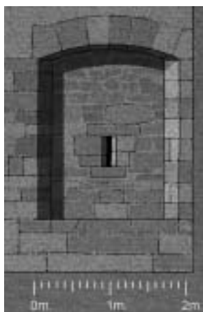
Figura 3. Para salvar el grueso del muro las saeteras se abren tras un lucillo cubierto con arco rebajado.
