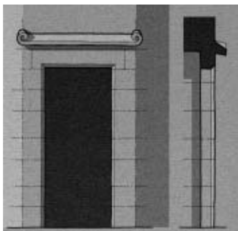
Figura 5. Alzado y sección de la puerta de acceso a la escalera de caracol.
