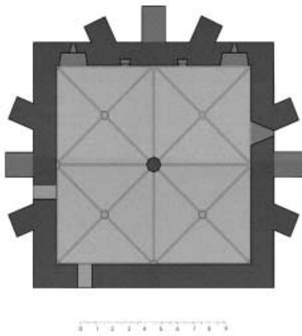
Figura 1. Se han incluido en la planta, en tono más suave, los supuestos contrafuertes centrales de las bóvedas de la cripta
