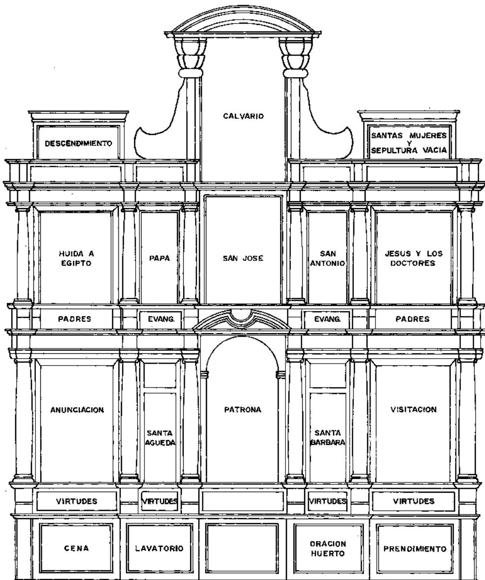
TRAZA DEL RETABLO MAYOR DE BIURRUN
