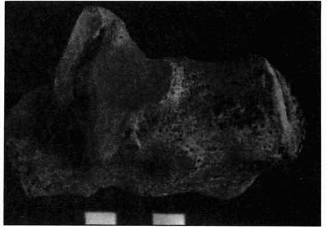
FIGURA 2. Calcaneo izquierdo.
