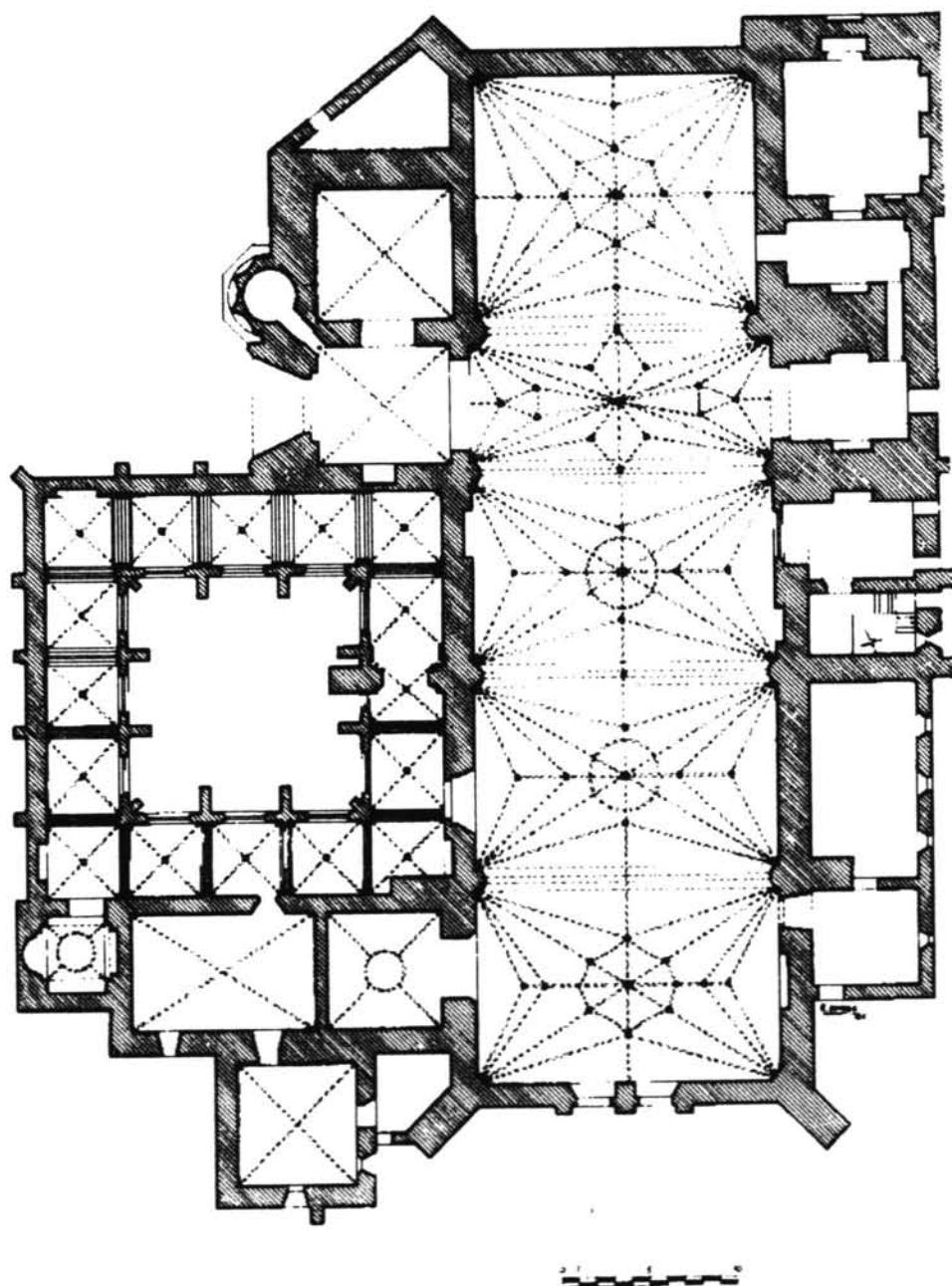
FIG. 1. Planta de la Catedral de Coria (Sánchez Lomba).
