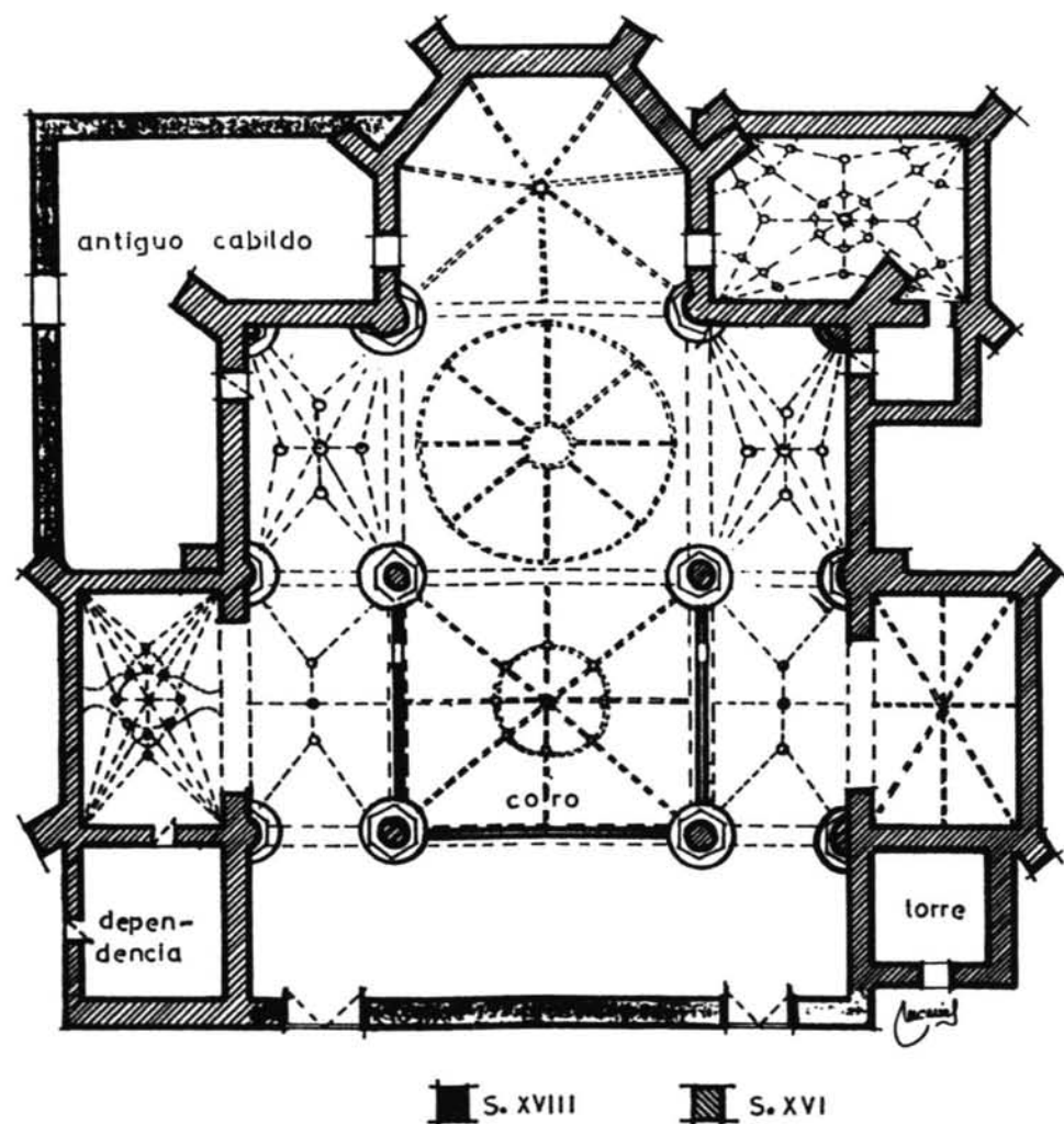
FIG. 2. Planta de la Colegiata de Villafranca del Bierzo (León) (Voces Jolías).
