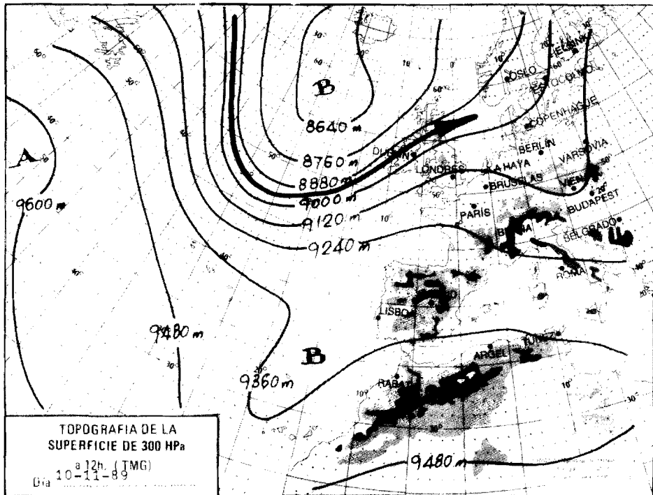
FIGURA 2. Una vaguada planetaria se formaliza a lo largo del meridiano 20°W. Al mismo tiempo que avanza ligeramente de Oeste a Este, va ganando amplitud, profundizando el aire frío hacia el Sur, alcanzando la región de Madeira.
