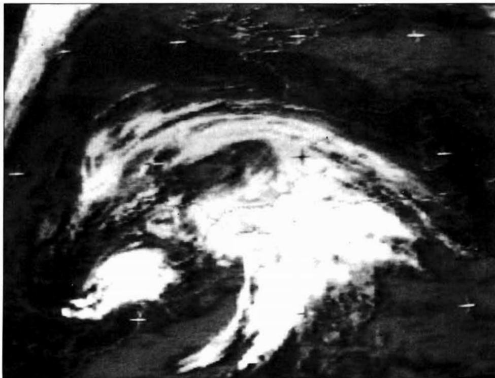
LÁMINA 4. La imagen infrarroja de METEOSAT, 20 h. 30' (T. M. G.) del 14/XI/1989, revela abundante nubosidad en la región levantina, Mediterráneo andaluz, Estrecho, Mar de Alborán, Marruecos. La presencia en niveles altos de un Chorro secundario del Sur acelera el disparo vertical de las células convectivas que adquieren un rápido desarrollo. Se forman núcleos de convección profunda sobre el área del Estrecho, Málaga, Mar de Alborán y Levante. Una gran tormenta arroja en la ciudad de Málaga 138 mm.
