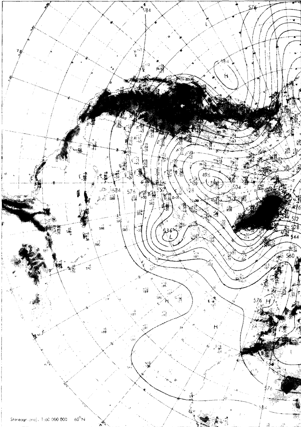
FIGURA 1. Condiciones dinámicas de la Circulación Norte, el día 15/XII/1989, a las 00 h. (T.M.G.).
