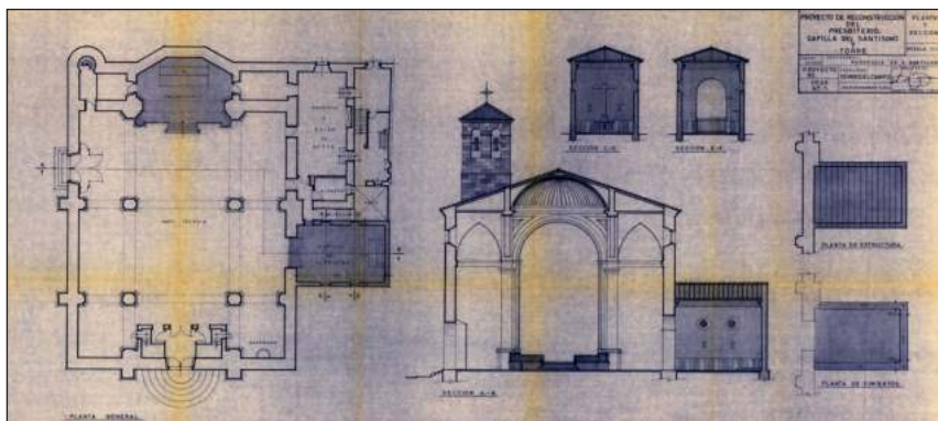
Fig. 10. Ramón Pajares Pardo. Proyecto de reconstrucción del presbiterio, Capilla del Santísimo y torre. Parroquia de San Bartolomé, Torredelcampo (1964). (FUENTE: Ministerio de Cultura y Deporte, Archivo General de la Administración, Fondo JNRTP (04)088.001, caja 52/04324, exp. s/n).
