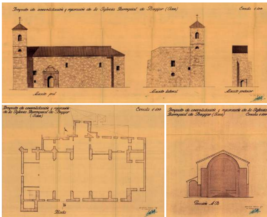
Fig. 4. Ambrosio del Valle Sáez. Proyecto de consolidación y reparación de la Iglesia Parroquial de Begijar (Jaén). Alzados. Planta. Sección A-B (1955) (FUENTE: Ministerio de Cultura y Deporte, Archivo General de la Administración, Fondo JNRTP (04)088.001, caja 52/04322, exp. s/n).
