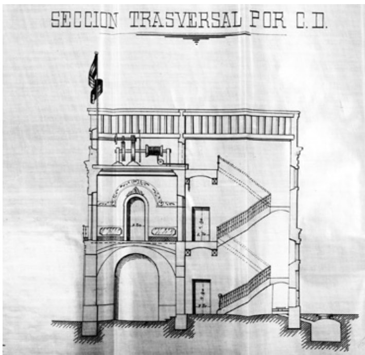
10. Proyecto planta baja y sección de la casa ayuntamiento, juzgado y cárcel provisional en Santiago de Carbajo. Emilio M. a Rodríguez (1885)
