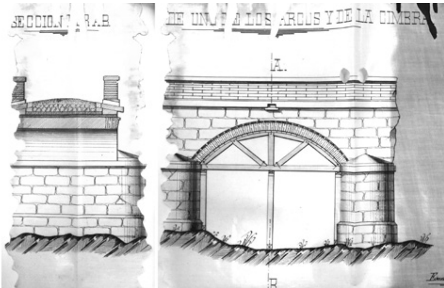
4. Sección del puente y detalle de uno de los arcos y de la cimbra
