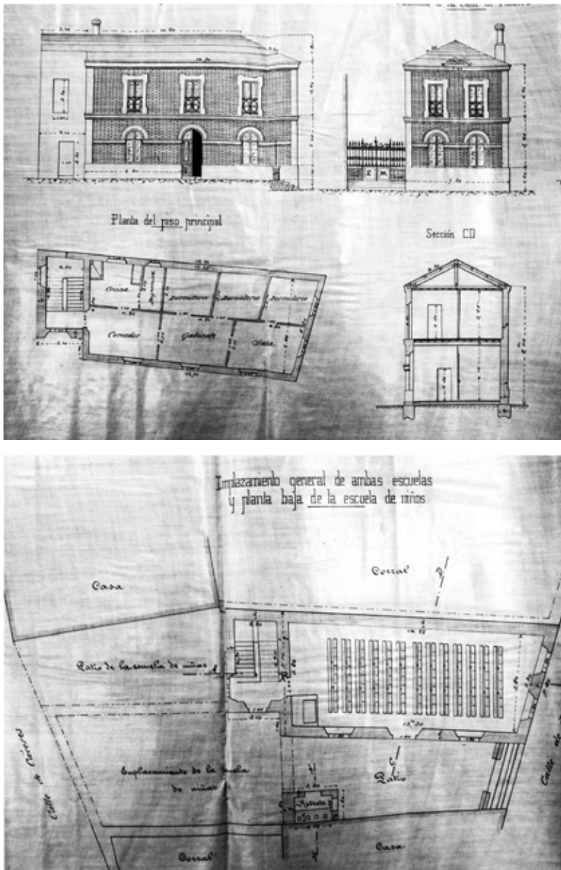
12. Proyecto de la escuela de niñas y casa del maestro en Moraleja. Emilio M. a Rodríguez (1901)
