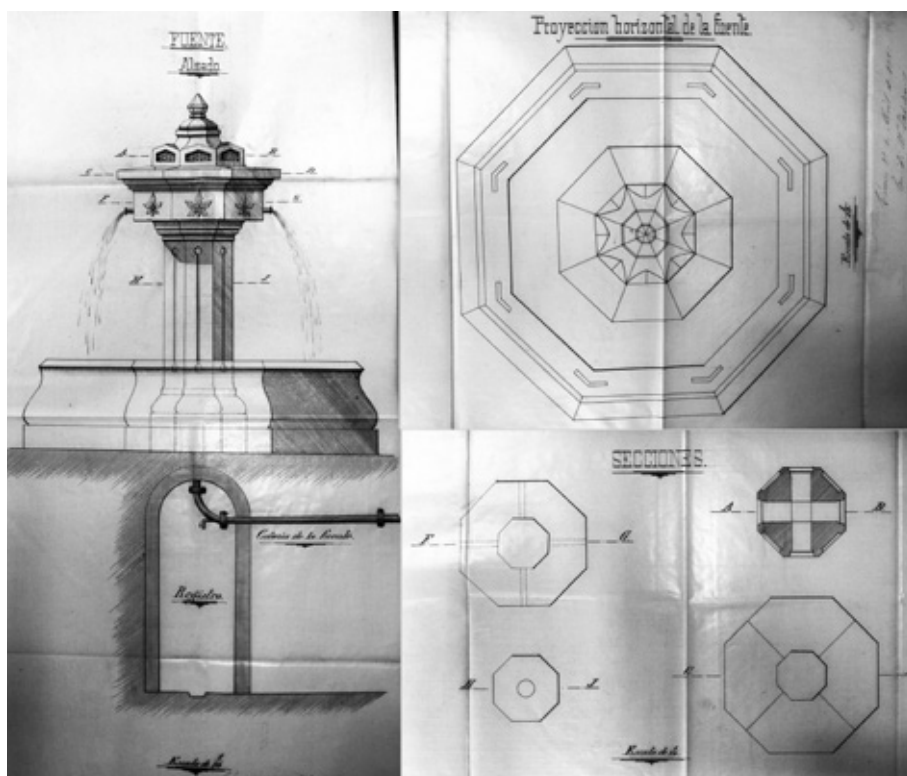
7. Proyecto de la fuente de la plaza de Santiago de Carbajo y secciones. Emilio M. a Rodríguez (1885)
