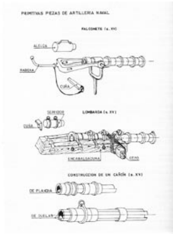
Fig. 7. Artillería Naval. Diagrama incluido en la obra del Almirante García Parreño Las armas navales españolas .
