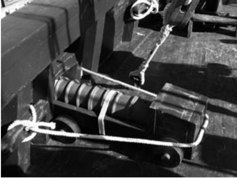
Fig. 8. Disposición de bombard reconstruida en el segundo puente de la nao “Santa María”. Fotografía Juan J. Toledo.
