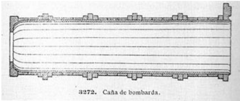
Fig. 5. Sistema de duela de una bombard de 30,5 cm. de calibre. Nº de inventario del Museo del Ejército 3272.
