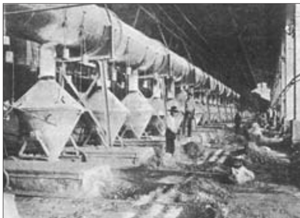
FIG. 4. Instalaciones de la Fundición de Plomo de Peñarroya (Horno Water-jackets de 20 toberas a la izquierda y Convertidores a la derecha) ( Estadística Minera... , 1911).
