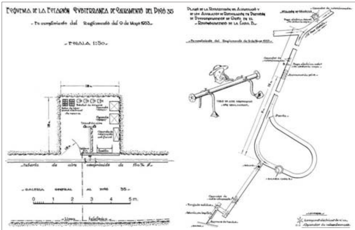
FIG. 8. Izquierda, esquema de una estación subterránea de salvamento; derecha, esquema de alumbrado y de distribución de aparatos de respiración ( Estadística Minera... , 1933).
