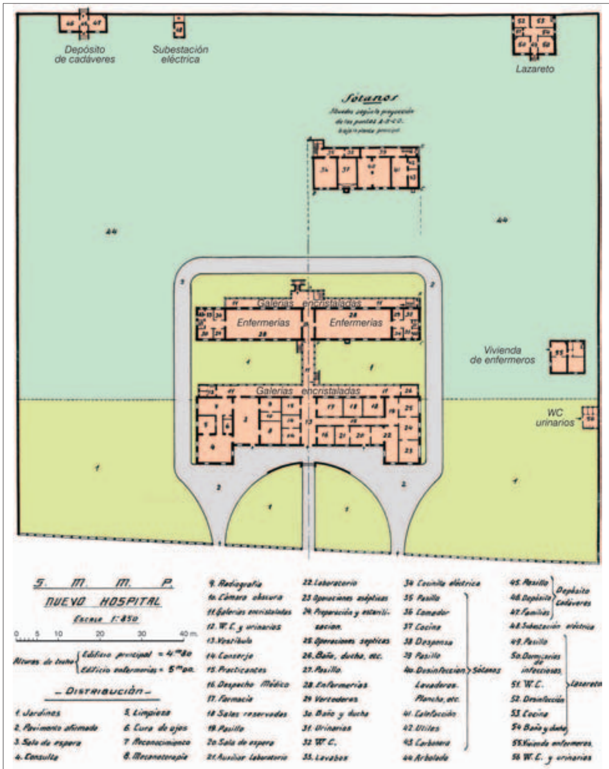
FIG. 11. Instalaciones del nuevo hospital de la S.M.M.P. (elaborado a partir de Estadística Minera y Metalúrgica de España ; 1929, págs. 266-269).
