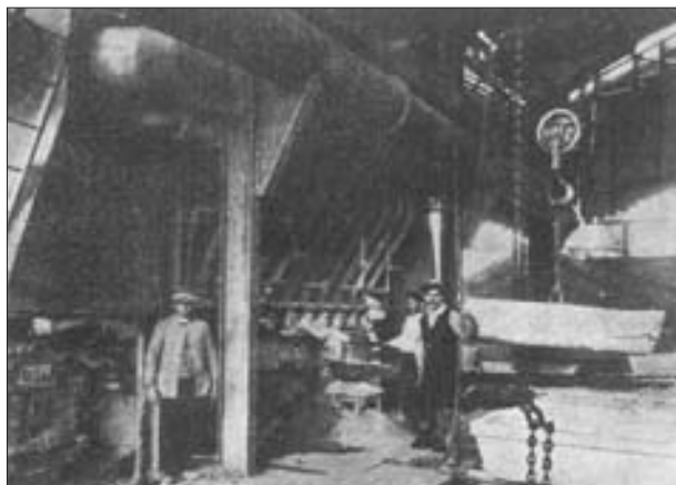
FIG. 4. Instalaciones de la Fundición de Plomo de Peñarroya (Horno Water-jackets de 20 toberas a la izquierda y Convertidores a la derecha) ( Estadística Minera... , 1911).
