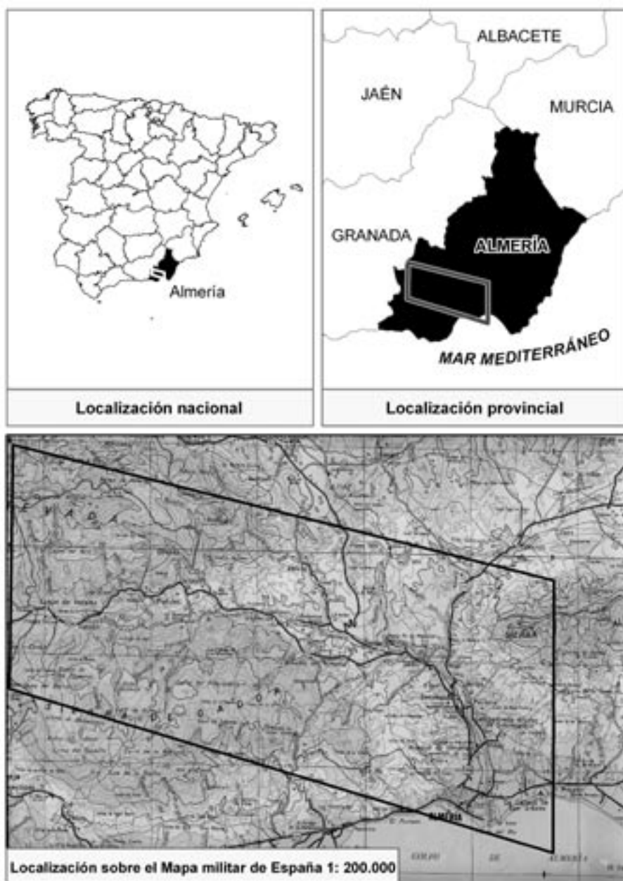
1. Situación del valle del río Andarax
