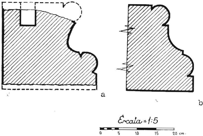
Fig. 2.—1. Sección basa Monasterio de San Pelayo. Oviedo.—2. Perfil basa de pilastra con casetones, en cabecera central. Iglesia de Santullano. Oviedo.
