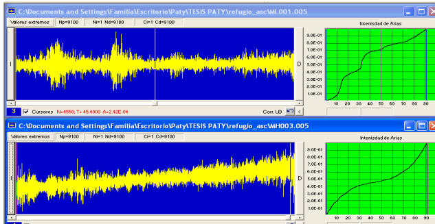
Figura 5. Registros originales de aceleración.
