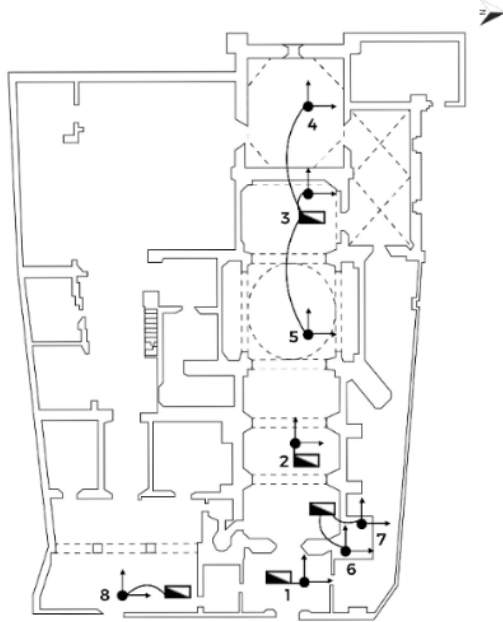
Figura 2. Croquis de la planta arquitectónica con la ubicación de los sensores. Editada por Soto, H. (2021).
