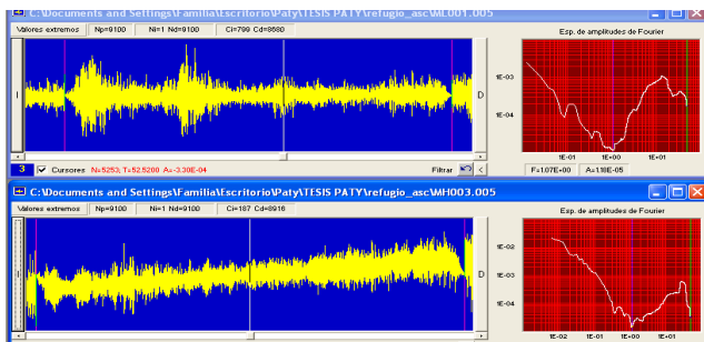
Figura 7. Espectros de Fourier donde se muestran las frecuencias de corte.
