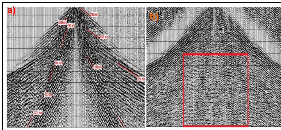
Figure 2. Tir sismique, a) avant filtrate ; b) après filtrage du ground roll
