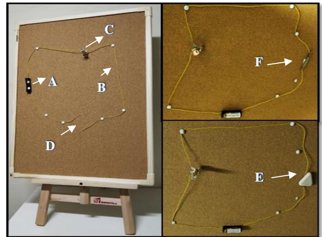
FIGURA 1. Quadro expositor do circuito elétrico simples. A- Suporte para pilha elétrica; B- Fio condutor de cobre; C- Bocal com lâmpada; D-Fio condutor rompido; E- Borracha; F- Pinça de metal.
