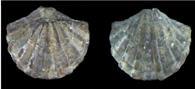
Fig. 1.- Gemmarcula crassicosta (Leymerie, 1869). Aptiense. Organyà. Medidas en el texto. Foto Carrasco.
