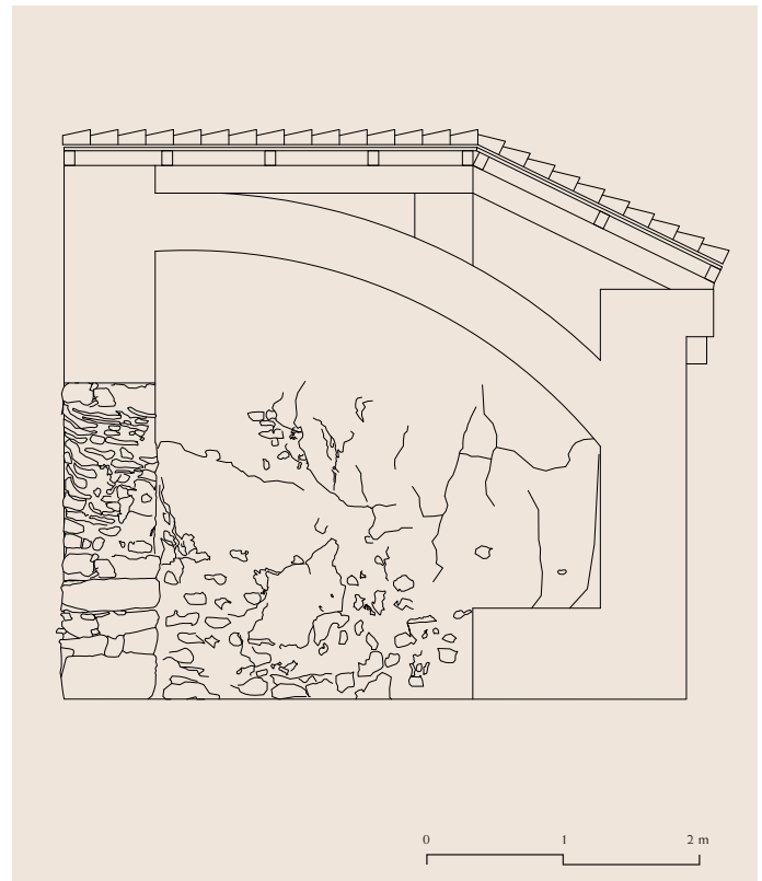
Sección transversal
