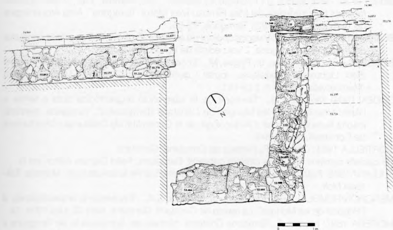
Planta de les restes de bestorre localitzades a l'Hospital de les Monges i paraments de muralla adjacents
