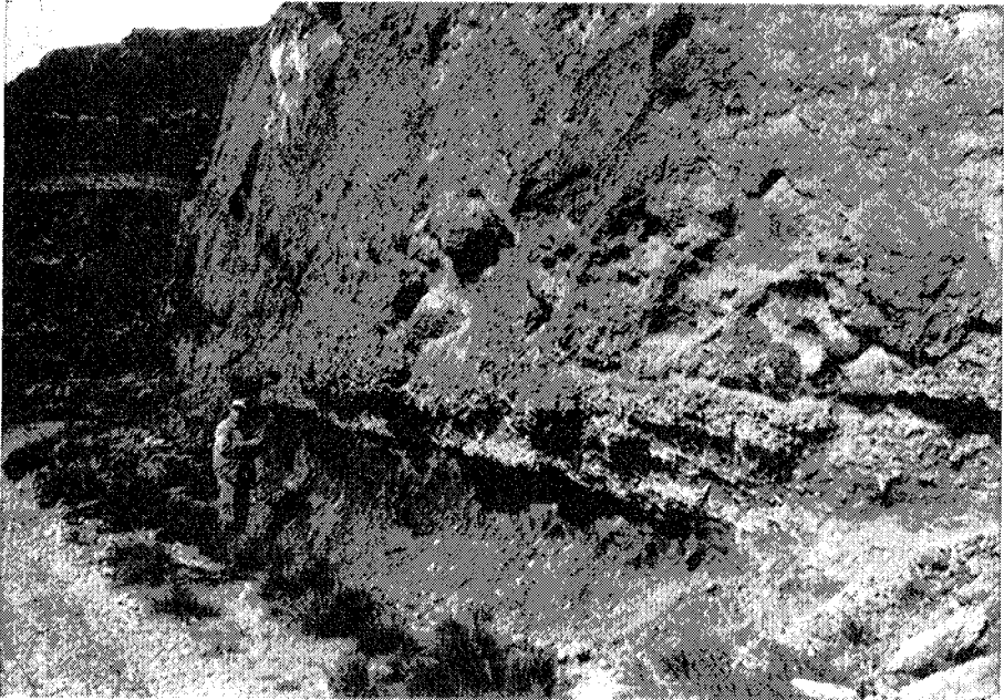
Fig. 7.— Afloramiento de la carretera local de Vúcar a Felix. Parte basal de la Formación Vúcar; areniscas con Heterosteginas y grandes Clypeaster , y bloques de dolomías perforados (←). El límite con el paleosuelo está señalado por un nivel de bioturbación. (Foto L. Delgado.)
