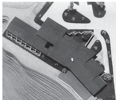
Figuras 14, 15, 16 e 17: Terceira versão. Planta, alçados e imagens da maquete. Pousada da Nazaré. Fonte: Arquivo Ruy Athougua.
