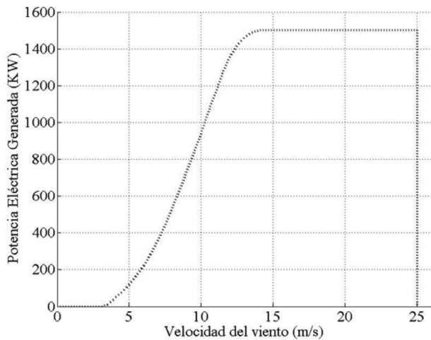
Figura 3. Curva de Potencia Generada
