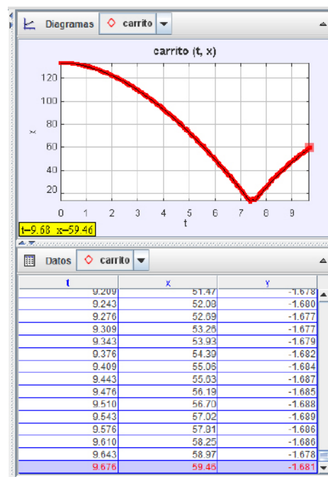
Figura 3. Gráfica y tabla de datos obtenidos a partir del video, usando Tracker
