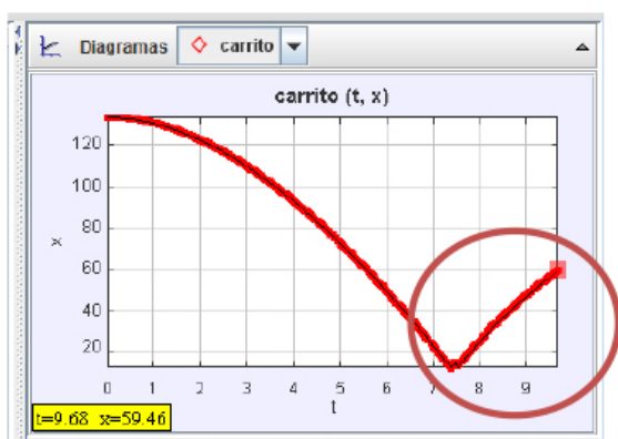
Figura 4. Información no útil identificada a partir de la gráfica construida Nota: Fuente propia de la investigación.
