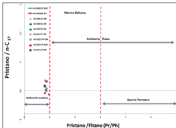
Ilustración 6. Relaciones Pr/Ph vs. Pr/nC17 de los crudos del área de estudio.
