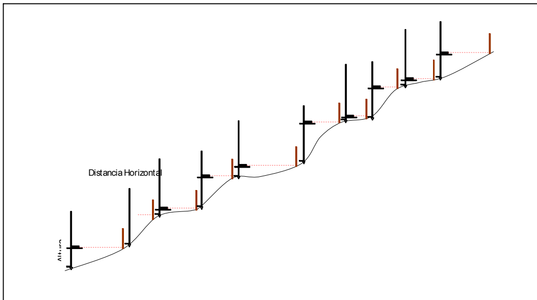
Figura 7. Distancia Horizontal Altura
