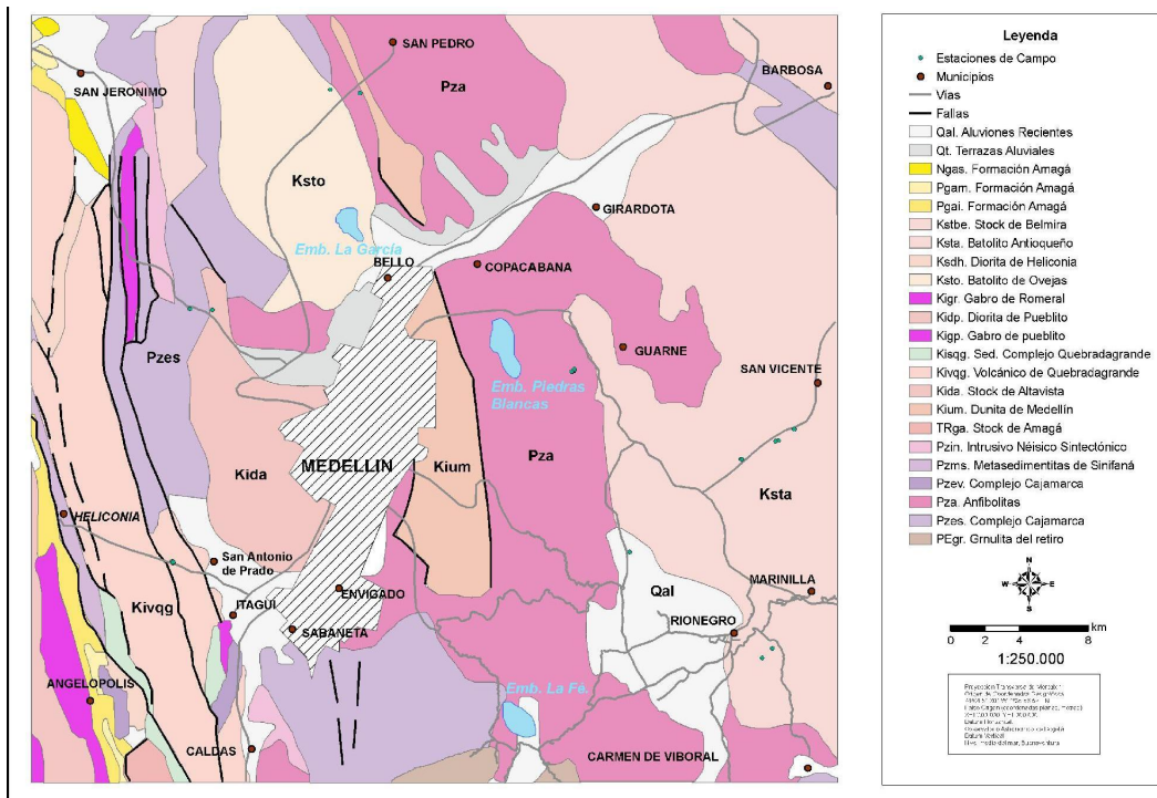
Figura 2. Mapa geológico.
