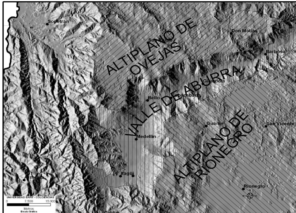
Figura 3. Geomorfología de la zona.
