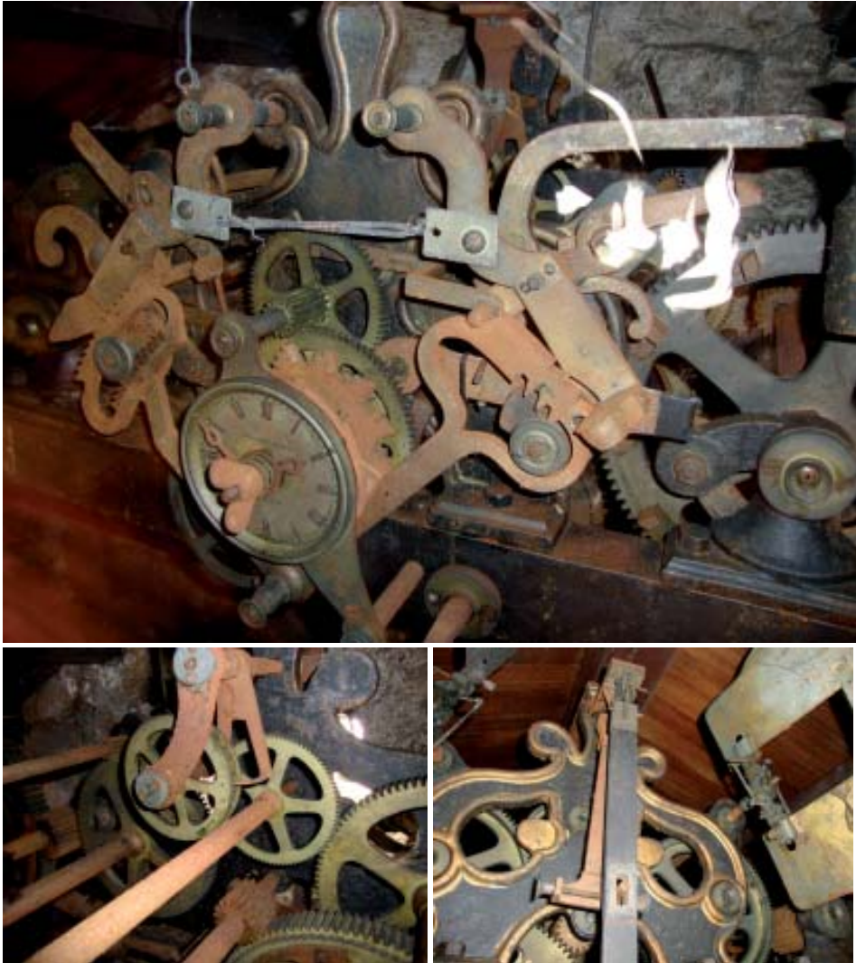
Diversas vistas de la máquina.
