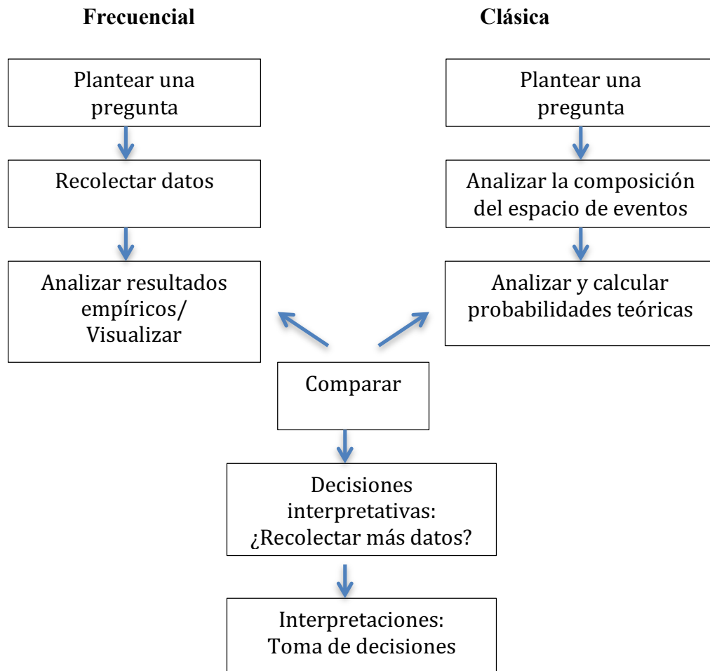
Figura 1: Un modelo para conectar las perspectivas frecuencial y clásica de probabilidad
