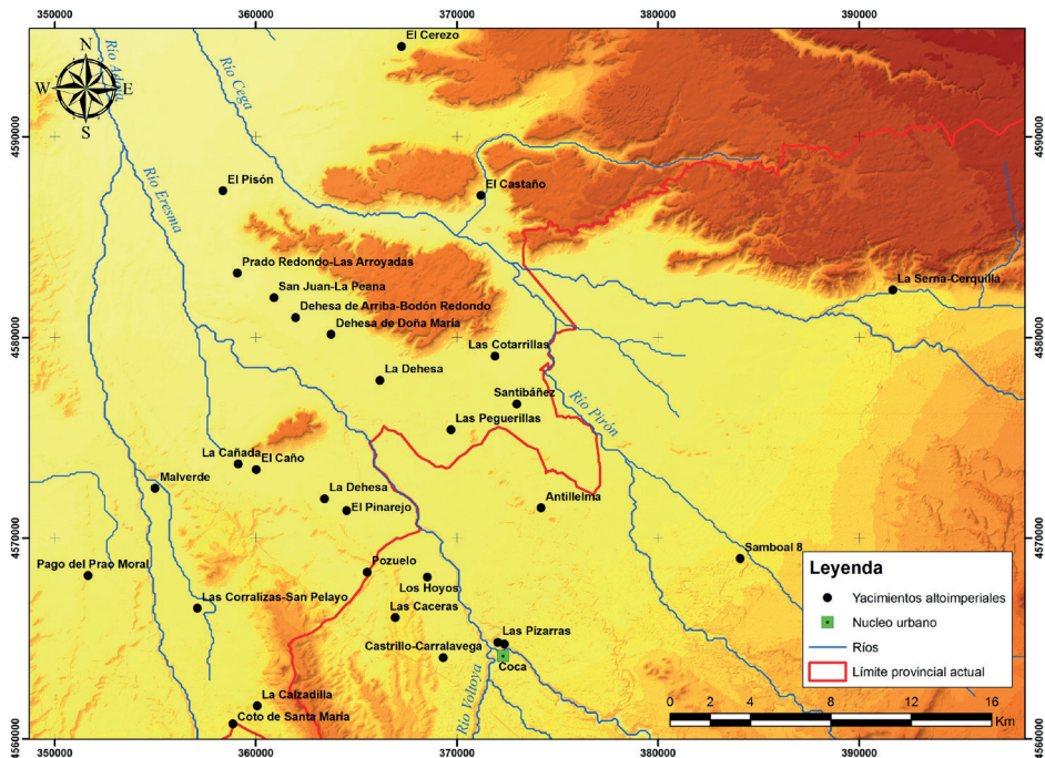
Fig. 10. Yacimientos romanos altoimperiales en Íscar y su entorno circundante. Se pueden observar los alineamientos señalados, especialmente el localizado al este del río Eresma.
