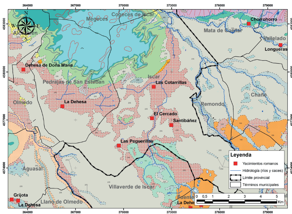
Fig. 2. Configuración geológica en el municipio de Íscar (Valladolid) y su entorno. Las áreas con trama cuadriculada, donde se localizan los yacimientos romanos, representan suelos formados por arenas pardas de origen poligénico, de potencialidad óptima para el laboreo agrícola. Cartografía de base: Mapa Geológico Continuo de España a escala 1:50.000 Raster (IGME).
