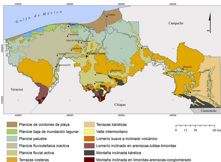
Figura 1. Paisajes geomorfológicos del estado de Tabasco.
