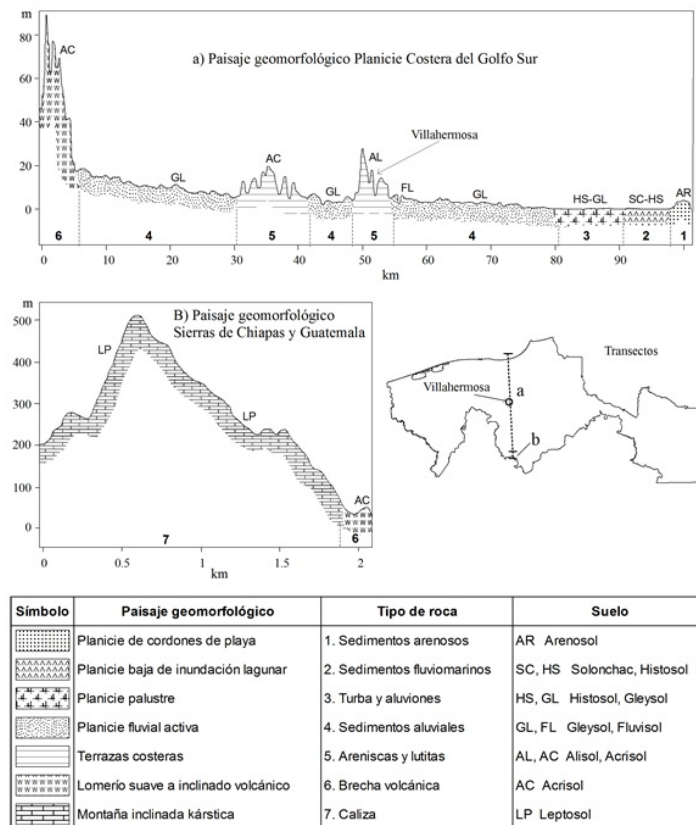
Figura 2. Paisajes geomorfológicos, rocas y suelos en el transecto Golfo de México-Sierra Norte de Chiapas.
