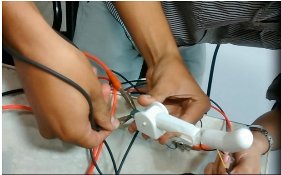
Fig. 9. Dedo impreso en PLA blanco Fuente: Autores.
