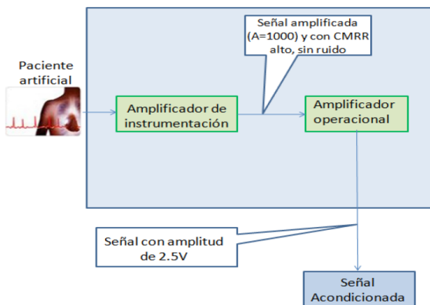
Figura 5. Acondicionamiento de la señal cardíaca. Fuente: Becerra, J. A. (2007). EGC móvil utilizando tecnología Inalámbrica . Bogotá, Colombia: Universidad Militar Nueva Granada.
