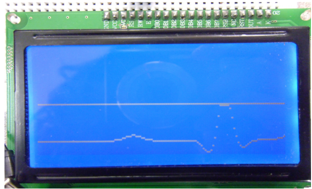
Figura 8. Visualización señal ECG en display gráfico.
