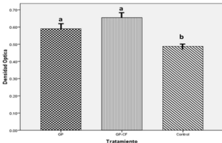
Figura 3. Valores de explosión respiratoria (OD) a las 8 h de animales desafiados con A. hydrophila y sometidos a concentración de 1000 \mu\text{g/L} de glifosato (GP), así como de su mezcla con Cosmoflux® 411F (GP-CF). Letras diferentes denotan diferencias estadísticamente significativas ( p < 0.05 ).
