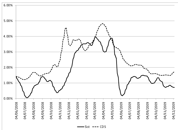
Gráfico 3. Componentes tendenciales del margen por riesgo sistémico títulos a cinco años y del CDS de Colombia a cinco años. Nota: Relación CDS vs. margen sistémico de cinco años Junio 2008 - Diciembre 2009.
