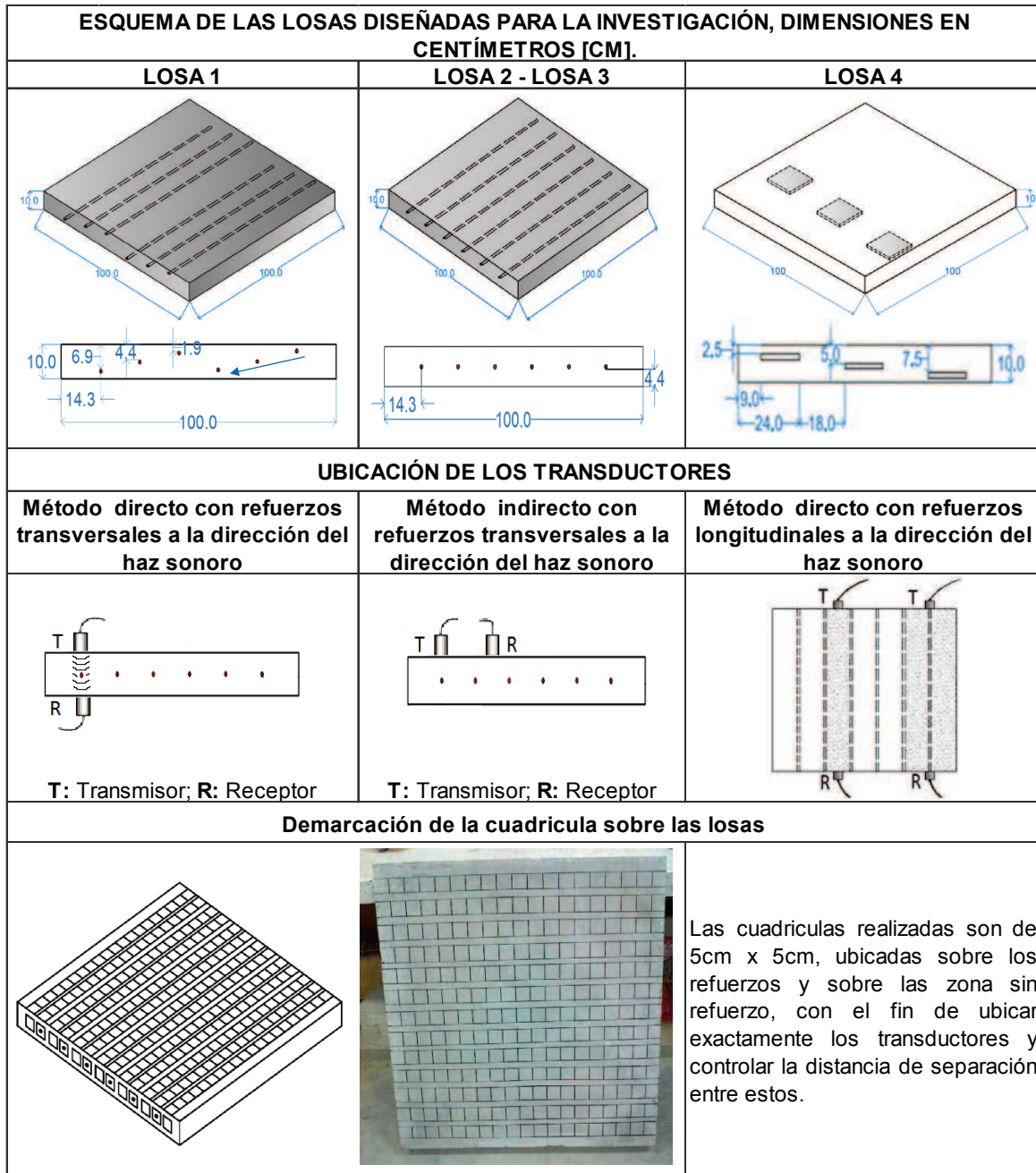
FIG. 2. Esquema de las losas diseñadas para la investigación y ubicación de los transductores; dimensiones en centímetros [cm].
