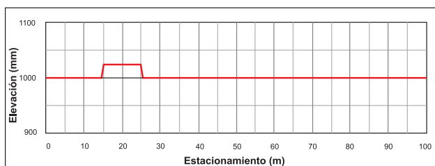
Figura 10 Simulación de un bache con un mal acabado superficial
