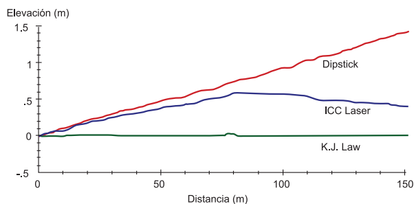
Variaciones aparentes de perfiles longitudinales utilizando diferentes equipos Figura 8
