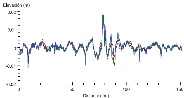
Los mismos perfiles de la figura anterior después del filtrado Figura 9
