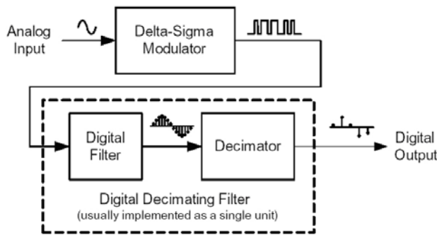
Figura 2. Arquitectura Conversor Sigma-Delta [14].
