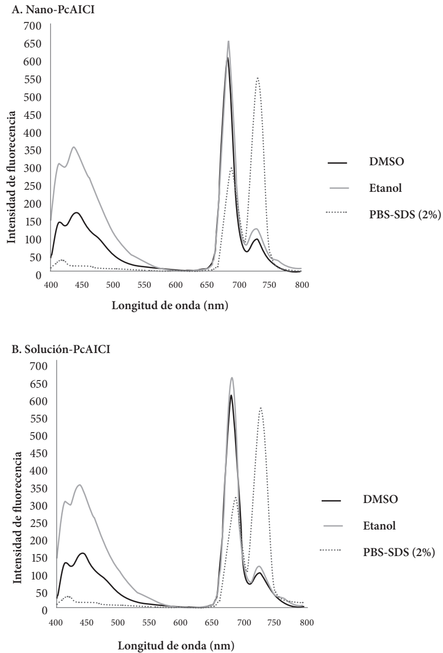
Figura 2. Espectro de emisión de la PcAICI en nano-PcAICI (A) y solución-PcAICI (B)
