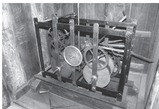
Fig. 3 Maquinaria de reloj fabricado por Daniel Torin, 1751 (explosión) (Foto: Victor Hevia).
