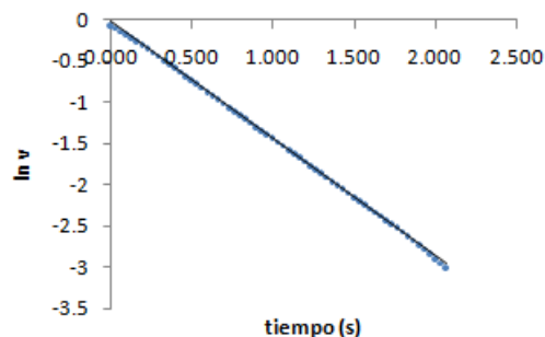
FIGURA 3. Gráfica de \ln v vs t , que permite determinar los parámetros del movimiento en el riel de aire horizontal.
