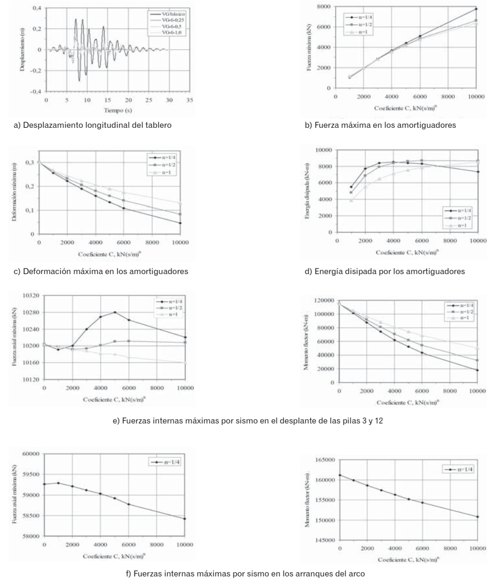
Figura 12. Respuesta sísmica del modelo VG ante un evento de fuente cercana
