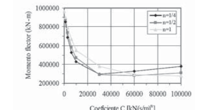
e) Fuerzas internas máximas por sismo en la base de las pilas 3 y 13
