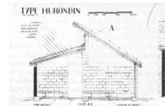
(Fig 2) Casas de refugio en adobe propuestas por LeCorbusier en 1940
