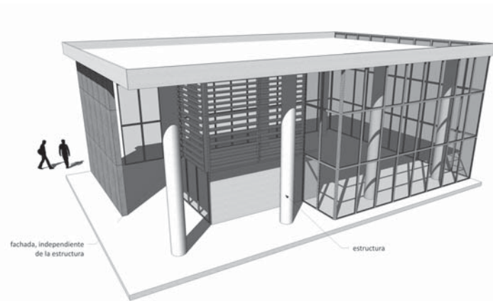
La fachada tiene orden independiente al de la estructura y se ubica libremente dentro del espacio. La ubicación de la fachada con respecto a la estructura es igualmente un recurso formal disponible.
