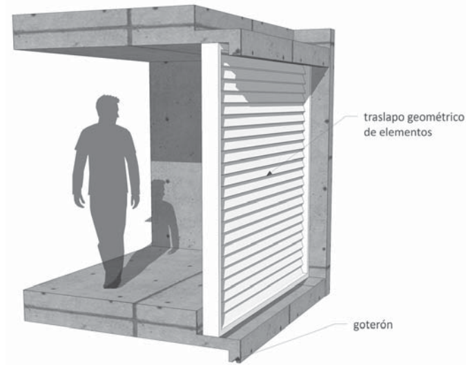
La geometría y el traslape sencillo son las herramientas básicas que el proyectista debe aplicar para enfrentar el problema del agua. El mejor ejemplo es el traslape utilizado en las persianas y en la parte superior e inferior de este ejemplo, donde siempre se busca que un componente solape sobre el otro.
