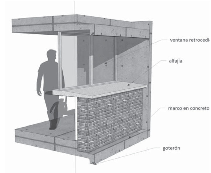
Adicional al solape de los elementos, como es el caso de esta alfajía con respecto al antepecho, generar fachadas profundas dificulta la llegada del agua a las juntas de la carpintería. Igualmente, un muro grueso de 25 o 37 cm, retarda la entrada del agua por capilaridad de forma eficiente, frente a un muro sencillo de 12 cm.
