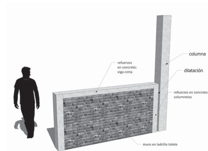
Un muro de fachada, reforzado con cintas de concreto, dilatado de la columna de concreto, garantiza el comportamiento independiente de los dos elementos.
