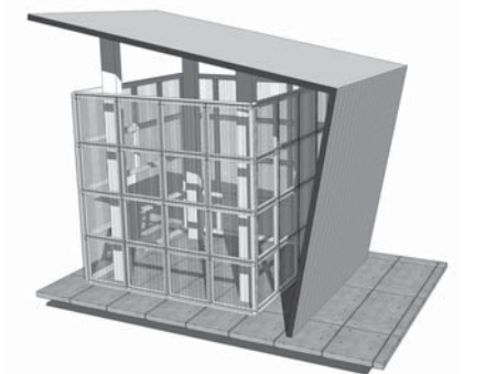
Esta solución es complicada ya que es difícil encontrar materiales que puedan solucionar el agua en dos direcciones contrarias; esto normalmente es posible con sistemas de panel tipo sandwich o con elementos continuos de concreto. La solución es válida para cubiertas planas e inclinadas.
