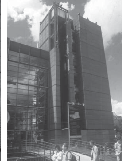
IRCAM, Renzo Piano, París. La práctica de "enchapar" el borde de los entrepisos para simular que la fachada es una piel continua ha sido muy criticada por diferentes académicos: problemas de estanqueidad, de decoloración y de estabilidad frente a empujes laterales.
