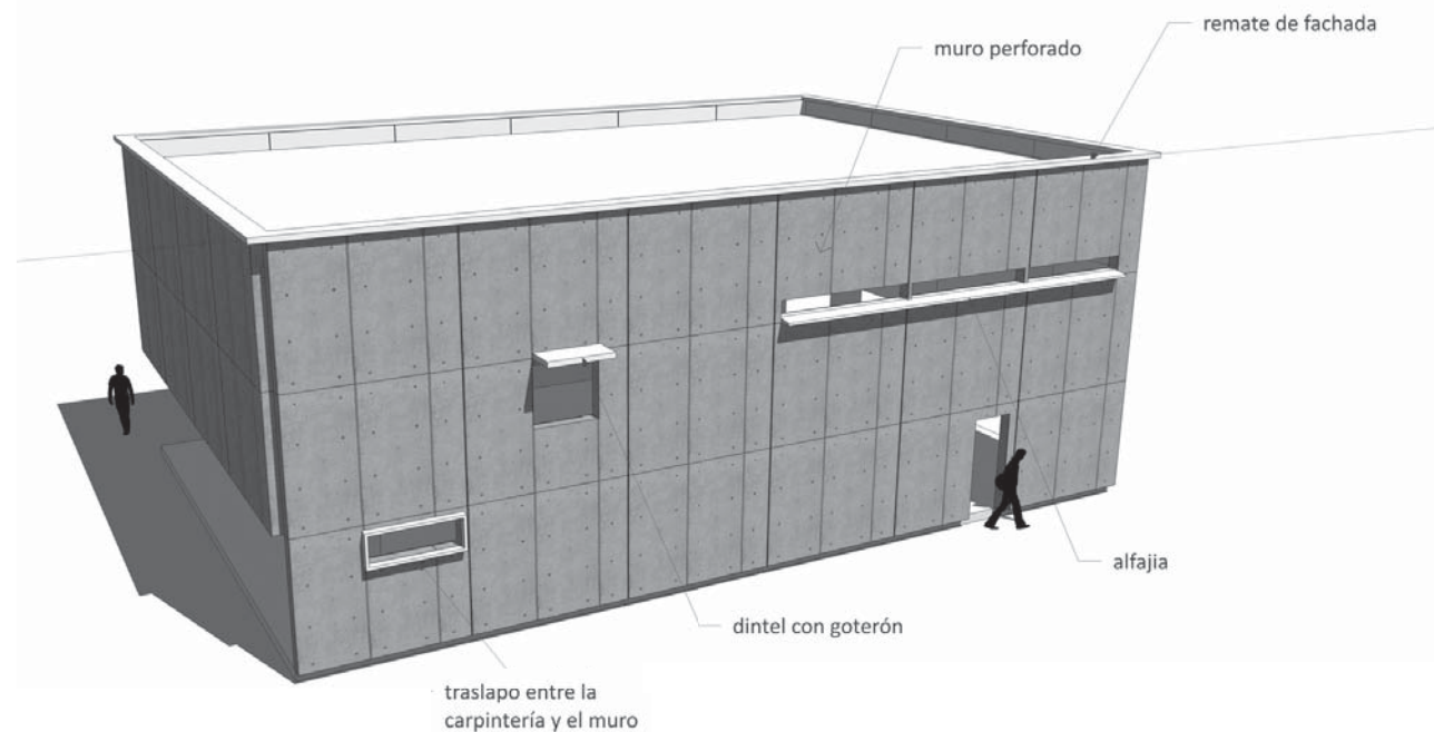
Una de las características más importantes de la arquitectura desarrollada en Colombia por arquitectos como Fernando Martínez, Rafael Obregón y Enrique Triana fue la utilización cortosos, goteros, alfajías, remates de fachada en concreto a la vista para controlar el movimiento del agua sobre la fachada. Esta es una práctica que desafortunadamente se ha perdido en el ejercicio convencional de la arquitectura actual.
