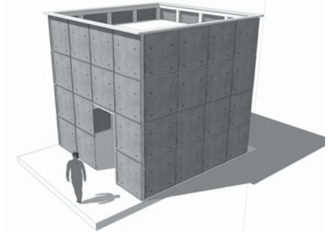
La cubierta no se percibe, dado el parapeto generado por la fachada; esto genera problemas de humedad en el trasdós de la fachada y la parte superior de la fachada queda totalmente expuesta, lo cual genera la aparición de un remate metálico o de un material de mayor impermeabilidad. La solución es válida para cubiertas planas e inclinadas.
