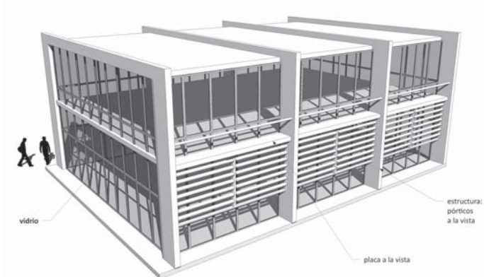
La fachada es un problema de carpinterías y cerramientos de diverso grado de transparencia, ya que la esencia del edificio la resuelve la estructura.
