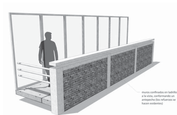
Antepecho en ladrillo cerámico confinado con elementos de concreto a la vista, modulados con el orden de la fachada
