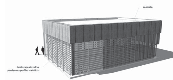
Las diferentes capas se pueden incorporar como parte del control de la incidencia del sol en el espacio interior.
