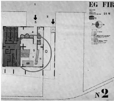
Figura 17. Plano del segundo nivel correspondiente a la tercera versión entregada en julio de 1962. Fuente: FLC, 16513a.
