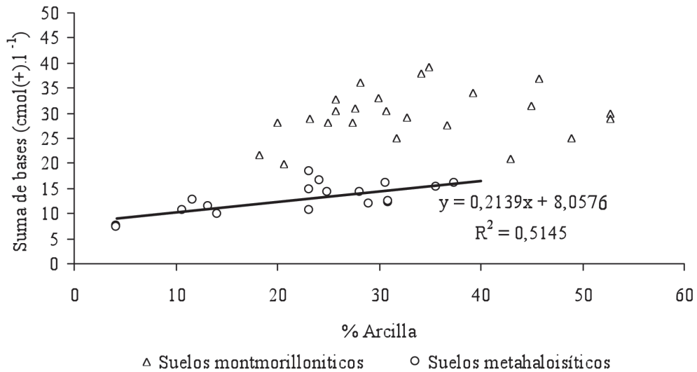
Fig. 3. Relación entre la sumatoria de bases y el % de arcilla en suelos de las familias montmorillonítica y metahaloisítica.
