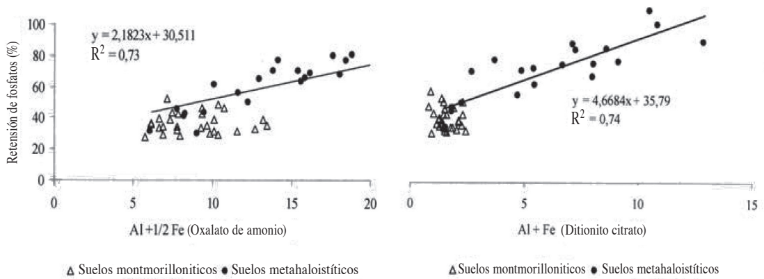
Fig. 5. Relación entre % de retención de fosfatos y la concentración de Al y Fe extraídos con Oxalato de amonio y ditionito citrato en suelos de las familias montmorillonítica y metahaloistítica.
